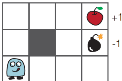
그림 13. 구현의 대상은 그대로 3×4 그리드 월드다. 평가할 정책만 무작위 정책에서 탐욕 정책으로 바뀐다. 출처: 원서 그림 4-15.
