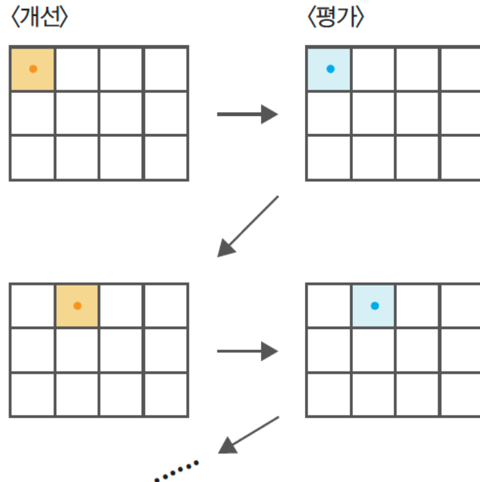
그림 4-21 각 상태에서 개선과 평가를 순차적으로 반복
