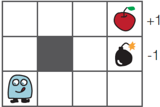
그림 4-8 3×4 그리드 월드
