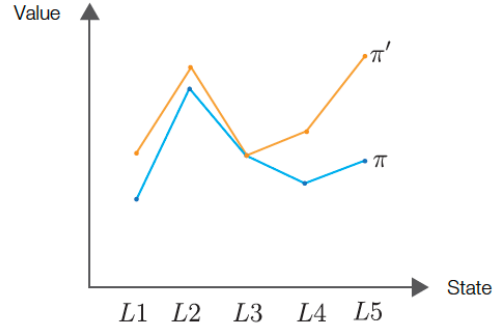
그림 2-11 모든 상태에서 v_{\pi'}(s) \geq v_{\pi}(s) 인 그래프
