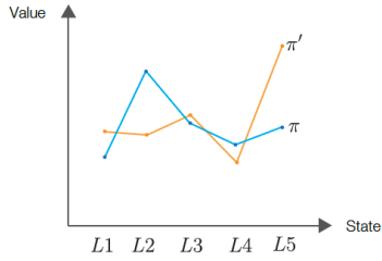
그림 2-10 정책 \pi 와 \pi' 각 상태에서의 상태 가치 함수 그래프(상태는 L1부터 L5까지 총 5개라고 가정)
