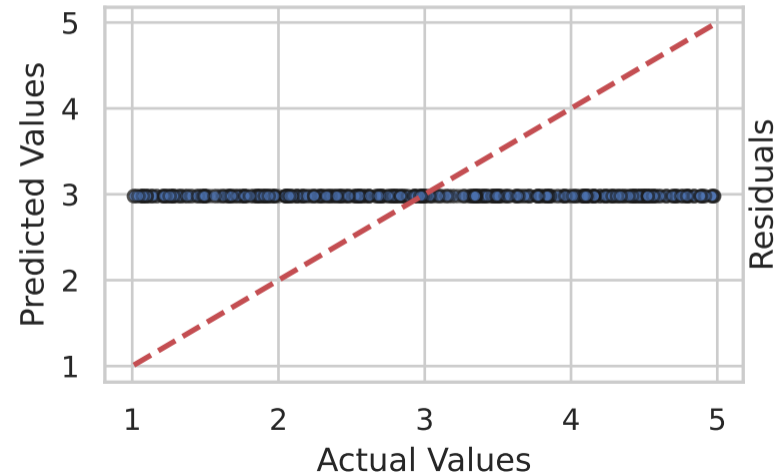
Actual vs. Predicted
