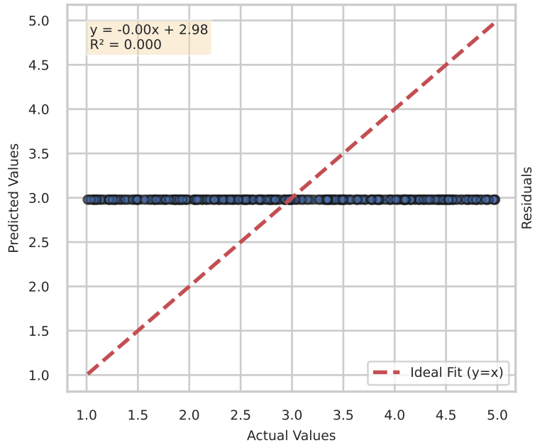
Actual vs. Predicted
