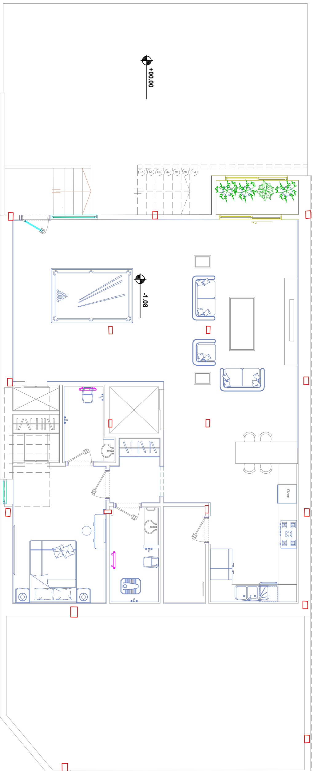
پلان معماری زیر زمین ۱-
