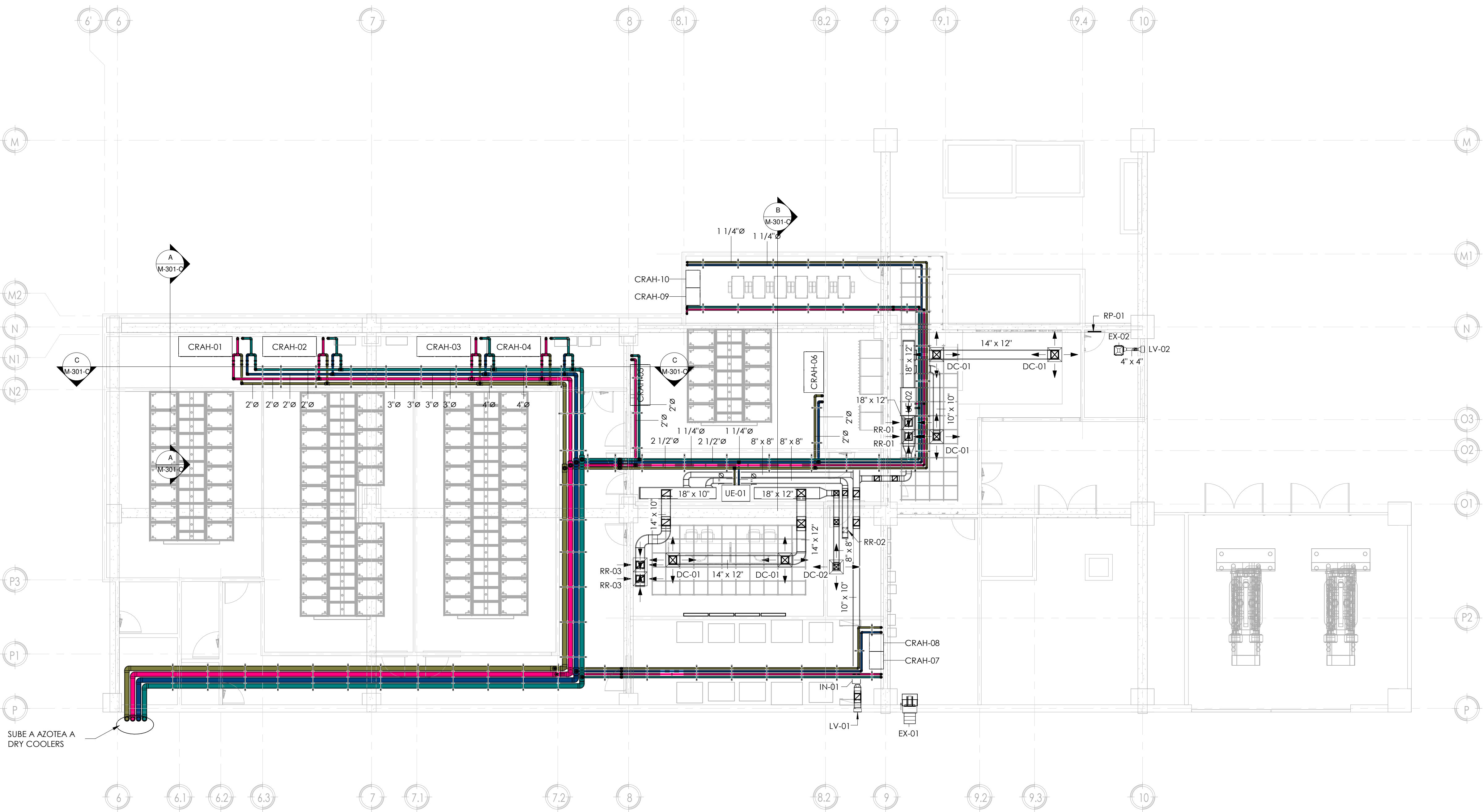
1 PLANTA DE AIRE ACONDICIONADO N1 ESCALA: 1 : 100
