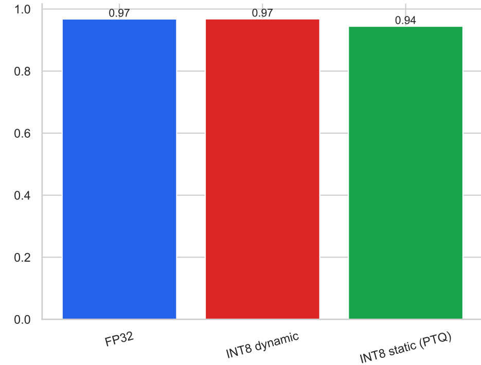
ROC-AUC
