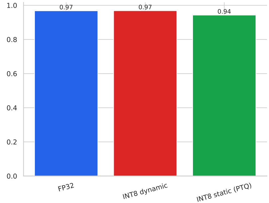
ROC-AUC
