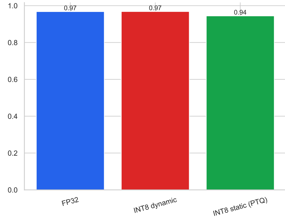
ROC-AUC
