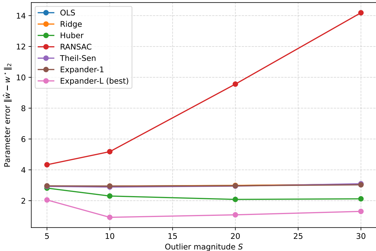
Parameter error vs outlier magnitude (alpha=0.3)
