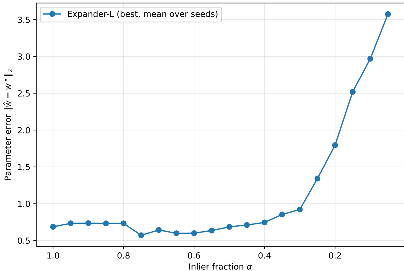
Expander-L parameter error vs \alpha (mode=uniform, n=5000, d=20)
