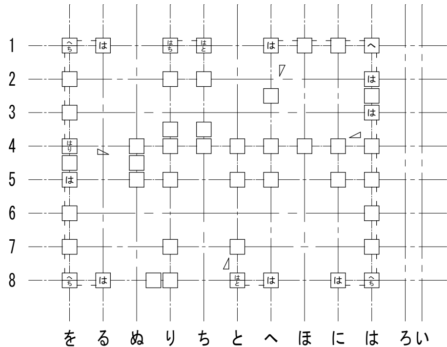
2階柱壁伏図
