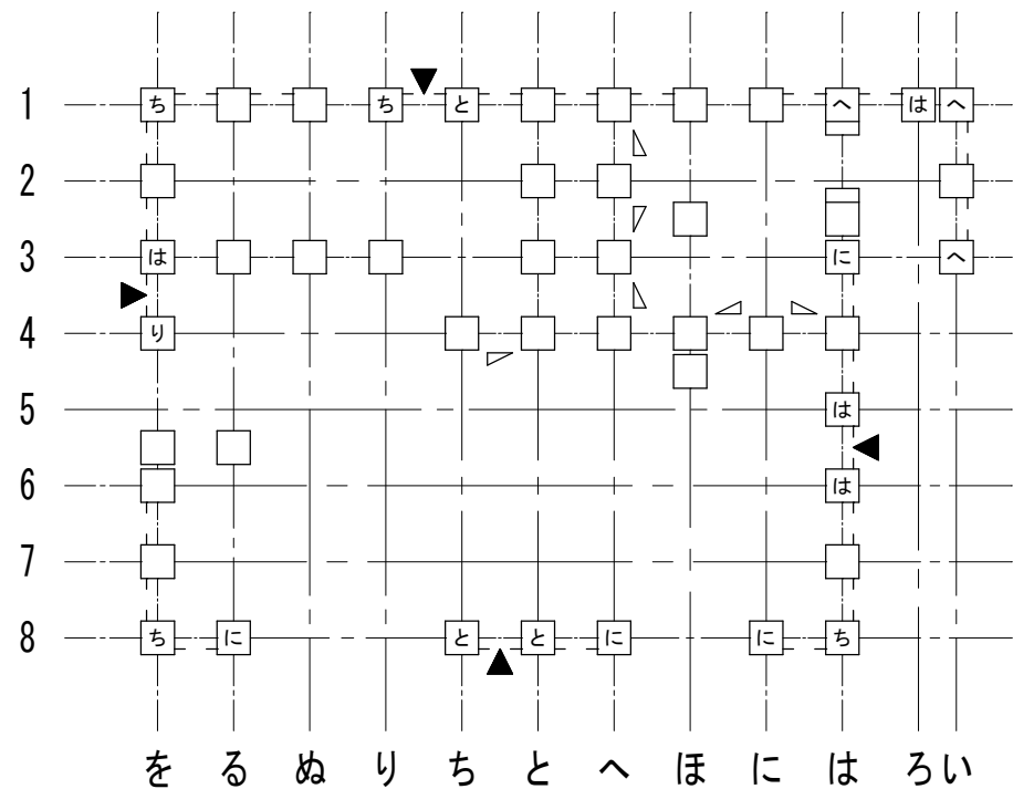
1階柱壁伏図
