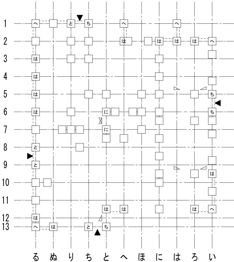
1 階柱壁伏図
