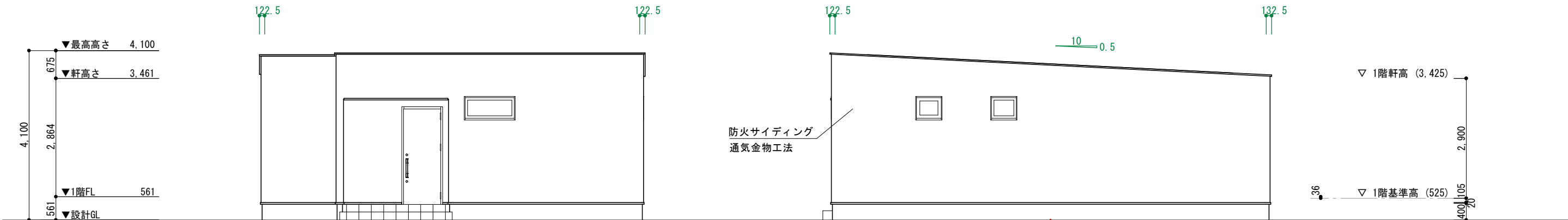
北立面図 S=1/100 北側立面図 S=1/100
