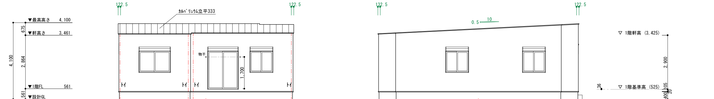
南立面図 S=1/100 南側立面図 S=1/100
