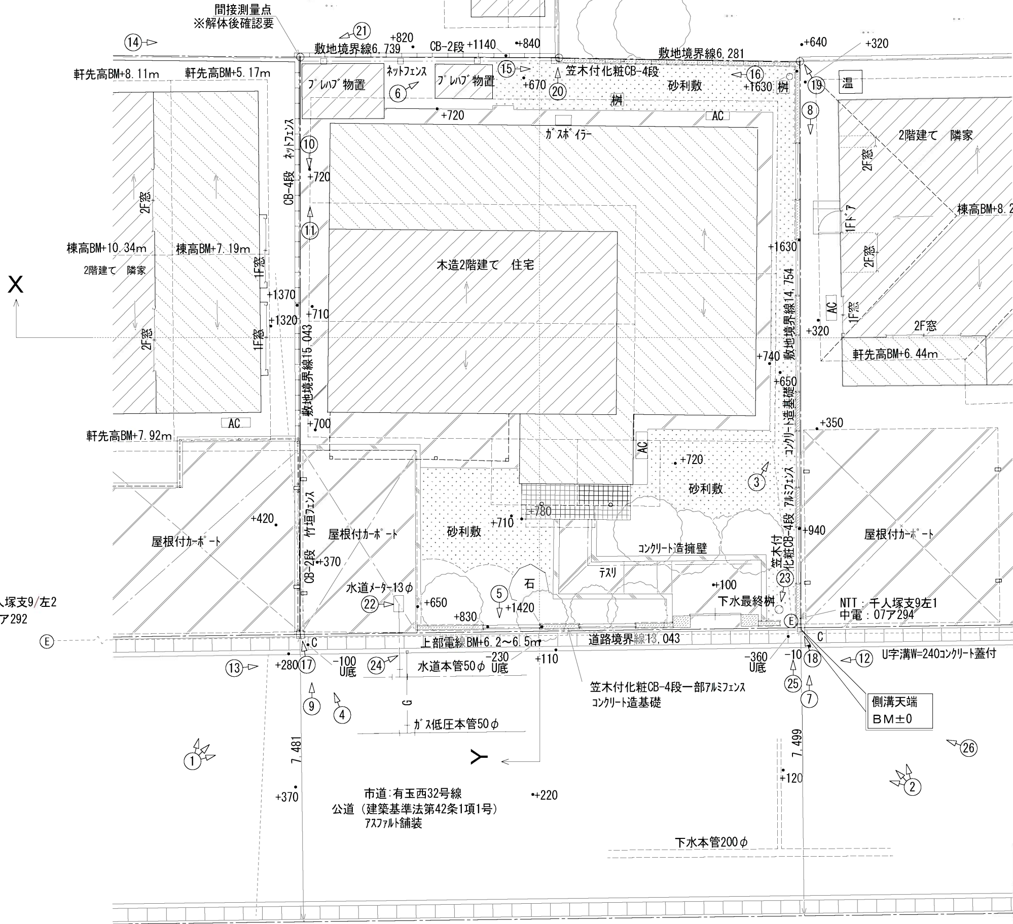
現況平面図 S=1/100
