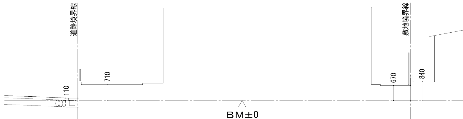
横断面図 (Y-Y') S=1/100
