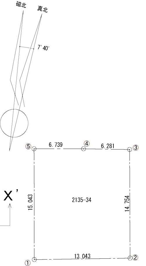
敷地面積求積図 S=1/300
