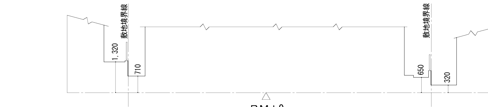
横断面図 (X-X') S=1/100
