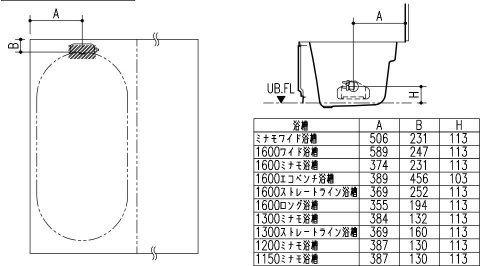
追いだき配管立上位置図
