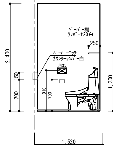
WC② 北面
