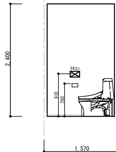
WC① 西側
