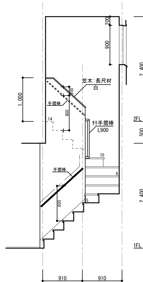
階段 南面
