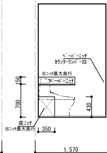
WC① 東側
