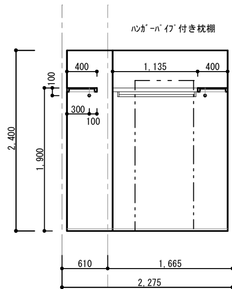
WIC 北面
