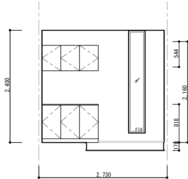
玄関 北面
