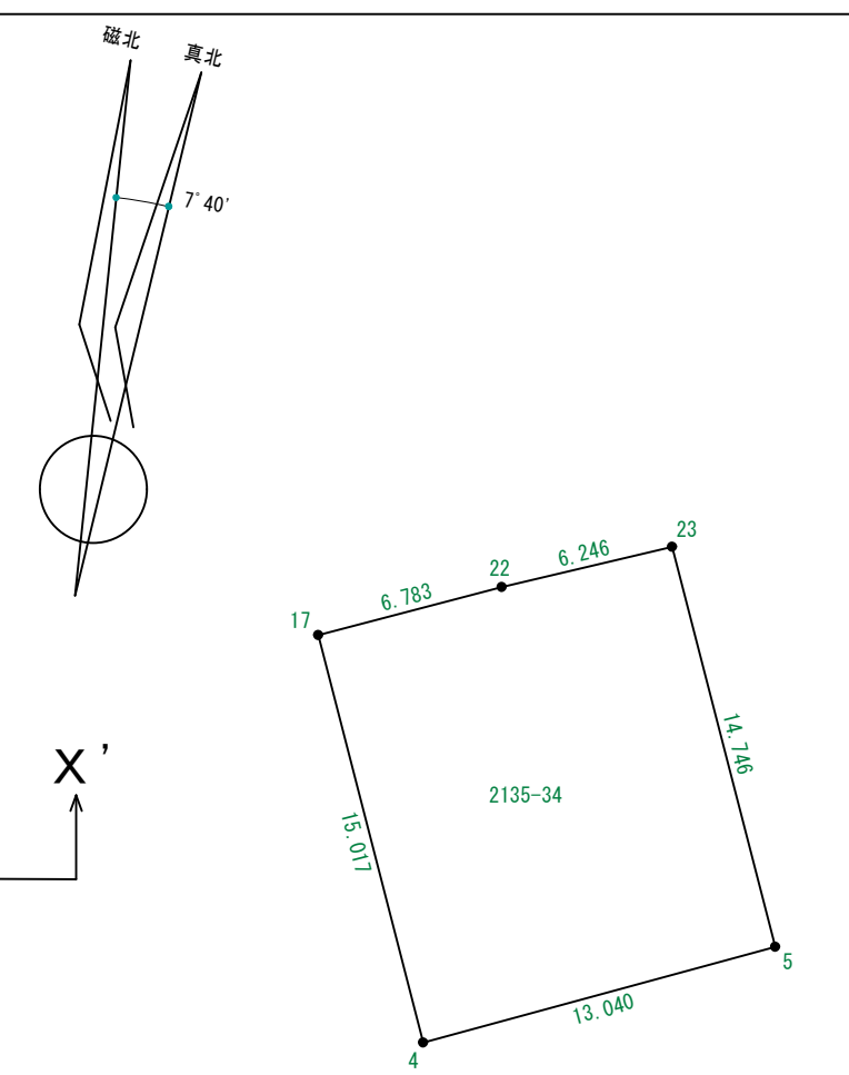
地 番 2135-34 N0 Xn Yn Xn · (Yn+1-Yn-1) 17 -138043. 243 -69916. 603 389005. 858774 4 -138057. 786 -69912. 858 -2254483. 645380 5 -138054. 372 -69900. 273 -1228269. 747684 23 -138040. 095 -69903. 961 1348237. 607865 22 -138041. 530 -69910. 040 1745121. 022260 合 計 -388. 904165 合 計 面 積 194. 4520825 地 積 194. 45 m 2
