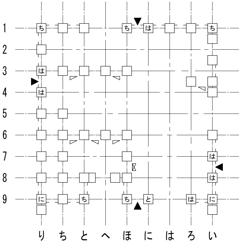
1階柱壁伏図
