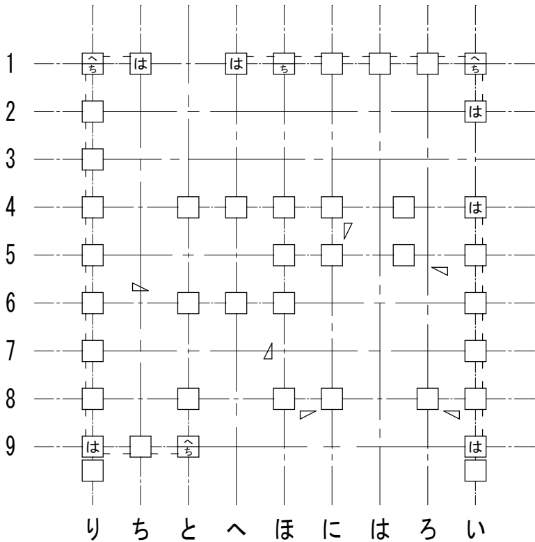
2階柱壁伏図
