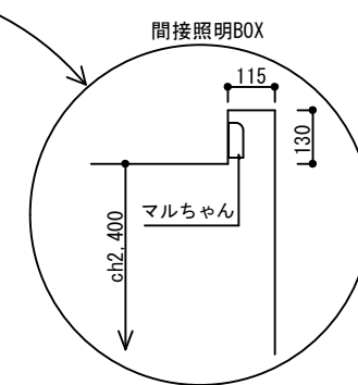
WC② 北面
