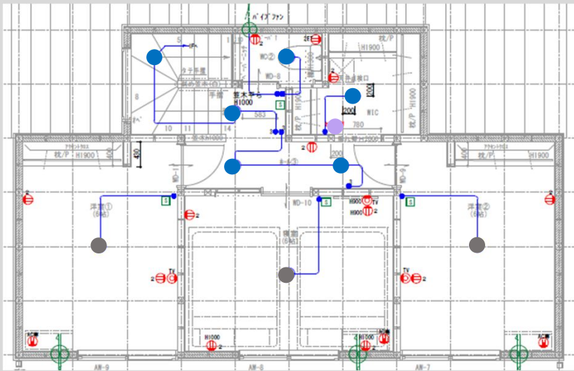
2階
