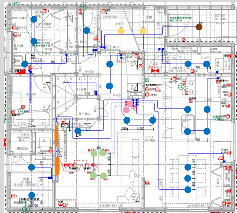
1階
