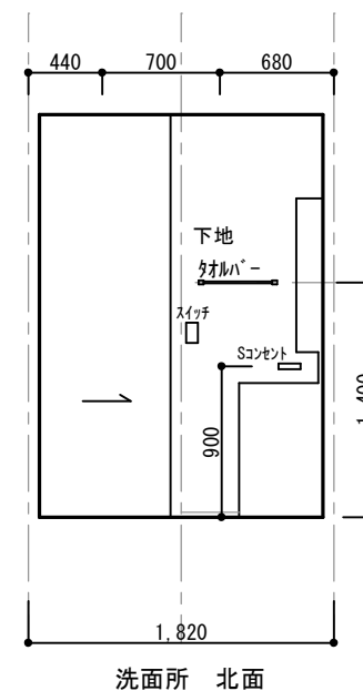
洗面所 北面
