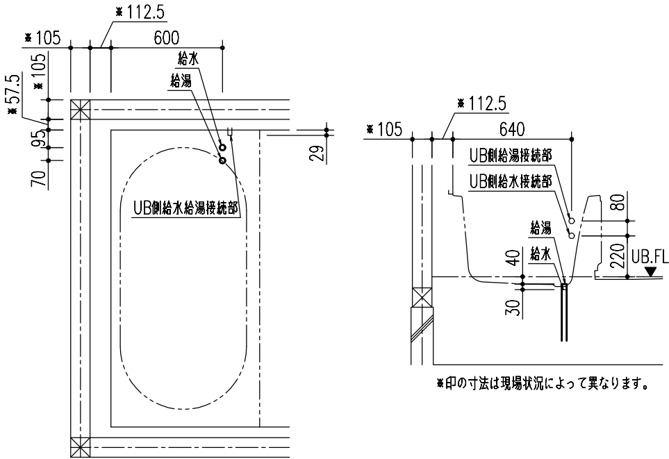
給水給湯配管立上げ位置 点検口止め
