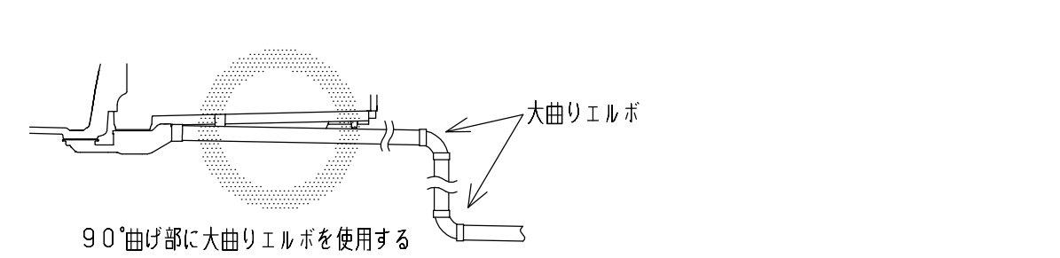
配管経路上に通気を設ける 配管径を拡張する 90°曲げ部に大曲リエルボを使用する ※浴槽排水時に排水口から「ゴボゴボ」と音が発生することがありますが、異常ではありません。
