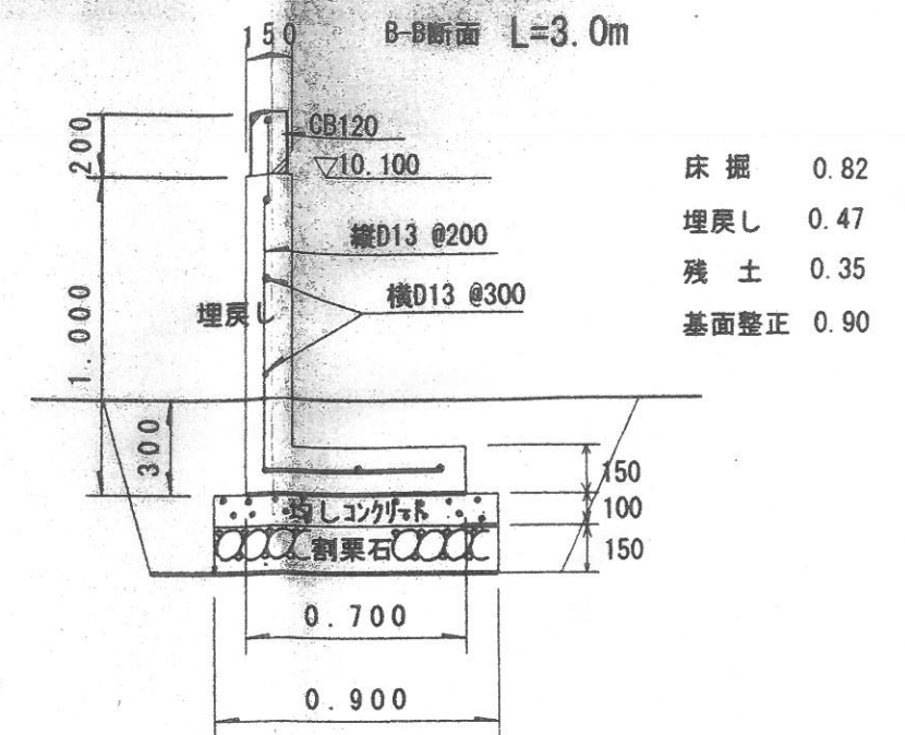
L型擁壁工 H=1000 S=1:25
