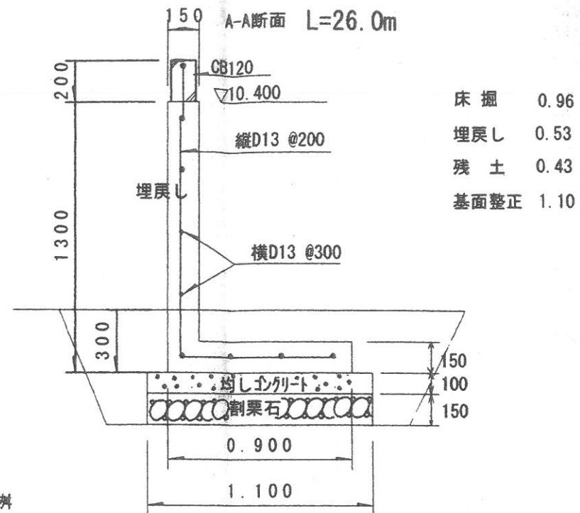
L型擁壁工 H=1300 S=1:25
