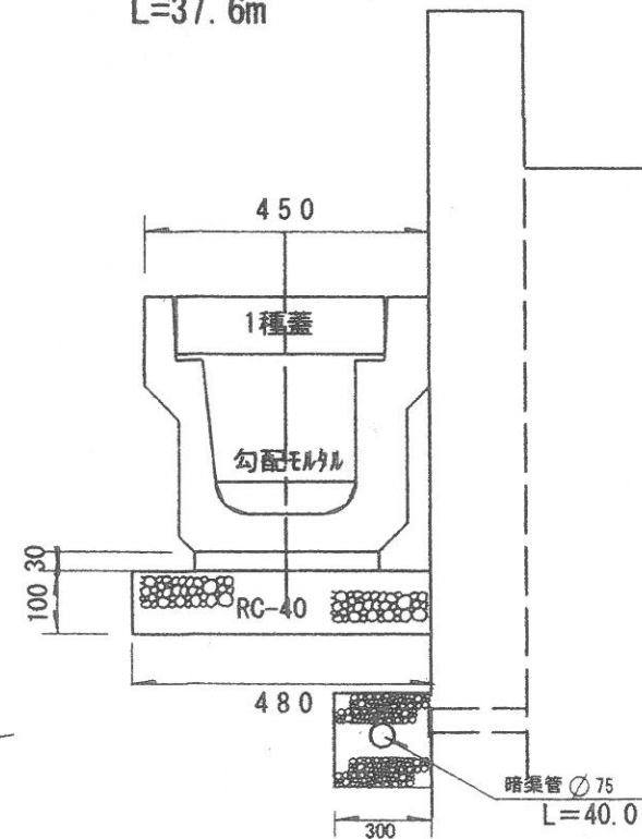
PU250 1種 D-D L=37.6m
