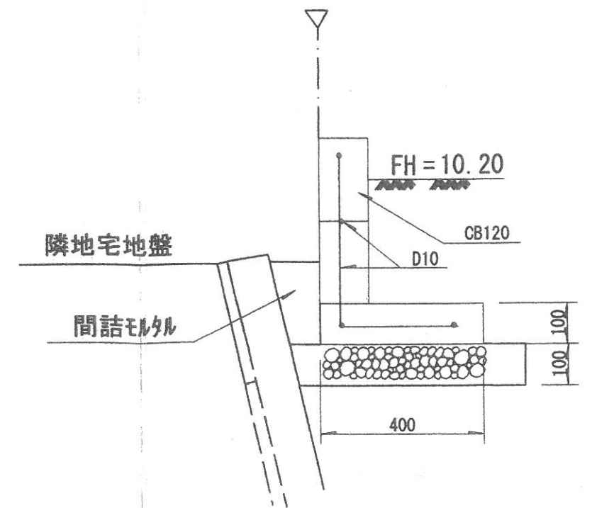
CB120積み 2段 C-C L=14.20m
