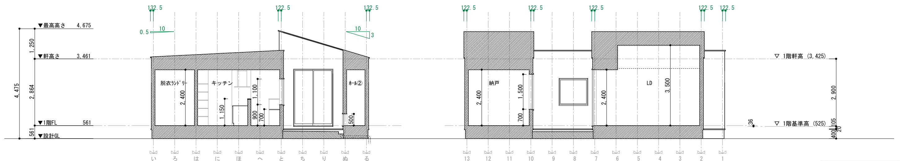
南側断面図 S=1/100
