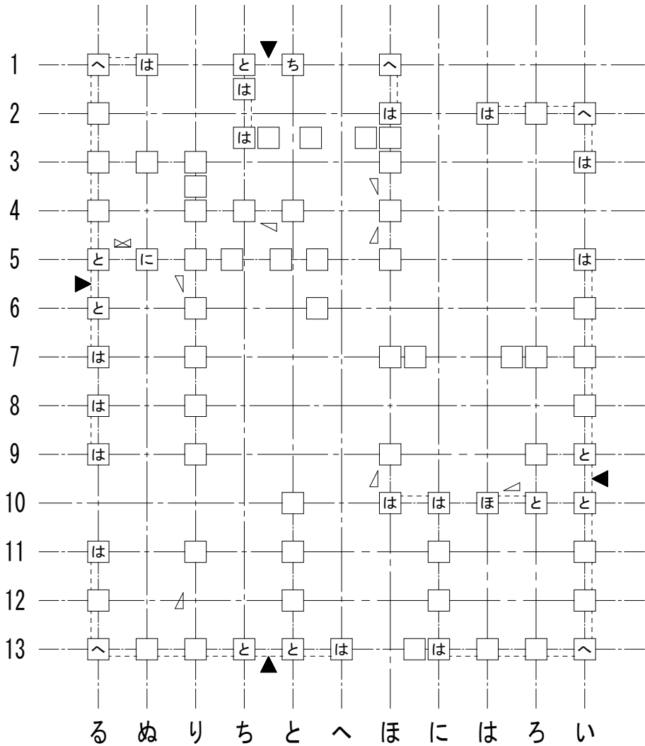
1 階柱壁伏図
