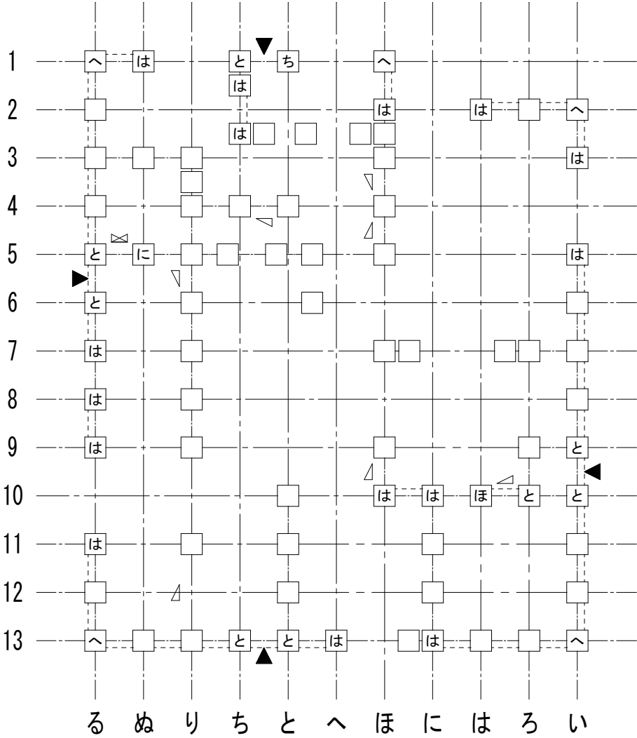
1 階柱壁伏図
