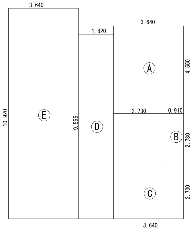
1階床面積図 S=1/100
