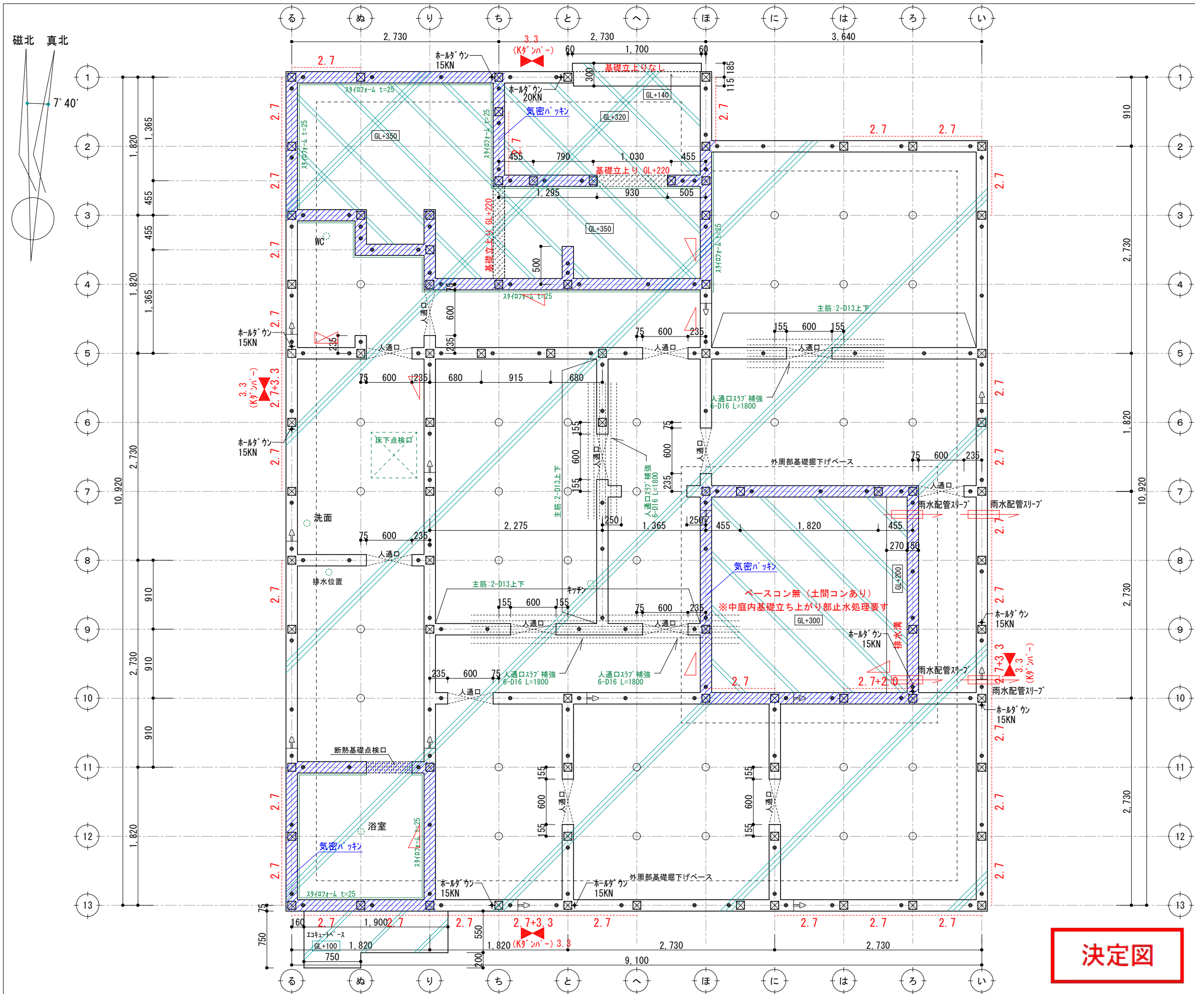
ホールダウン用アンカーボルト配置
