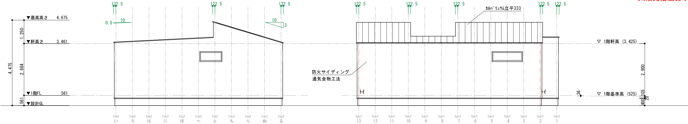
南側立面図 S=1/100
