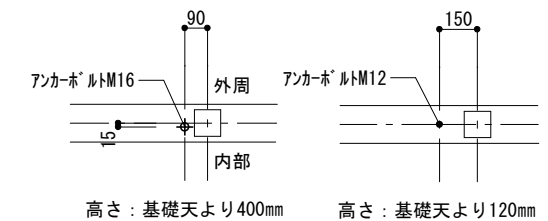
ホールダウン用アンカーボルト配置
