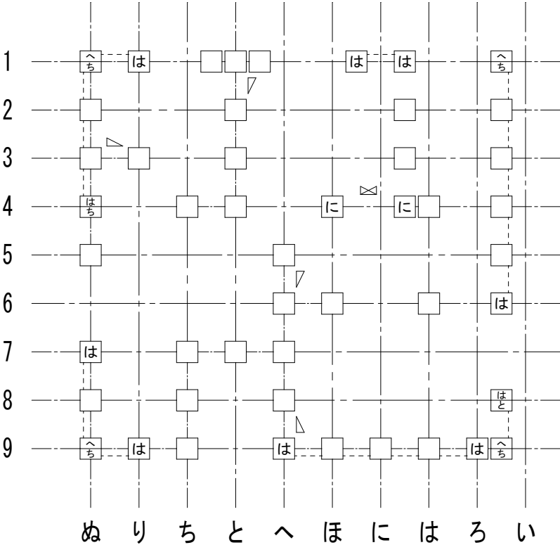
2階柱壁伏図
