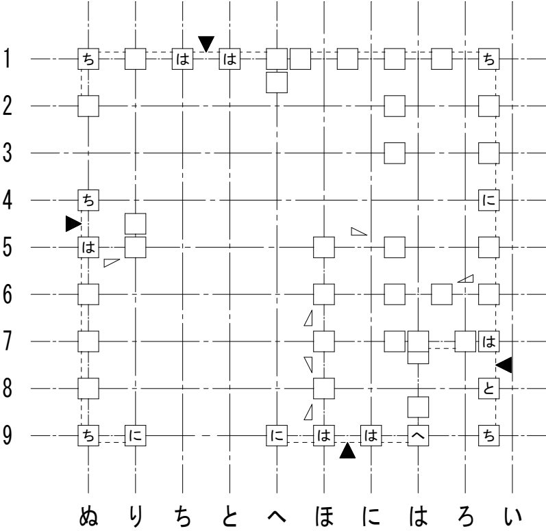
1階柱壁伏図
