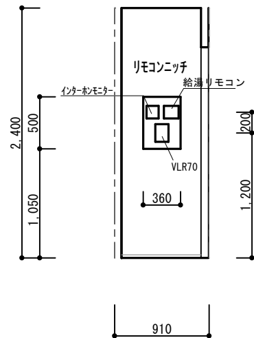
LDK 南面
