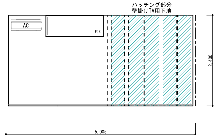
LDK 東面
