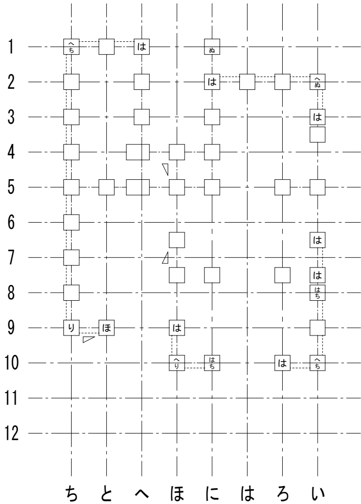
2階柱壁伏図
