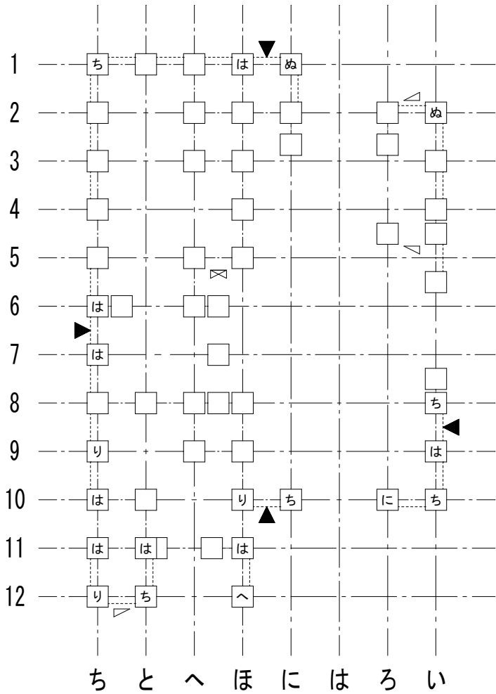
1階柱壁伏図
