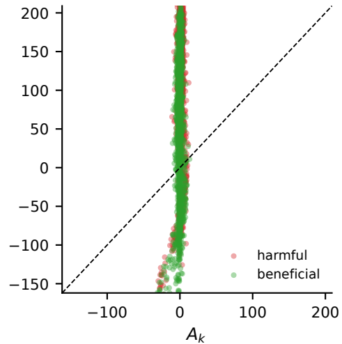
LunarLander
