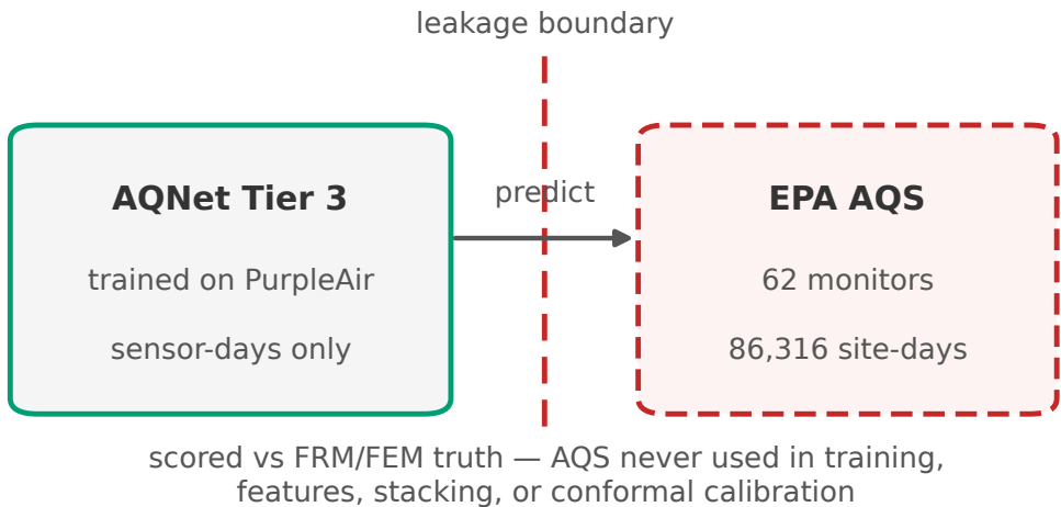
(d) external validation — EPA AQS FRM/FEM
