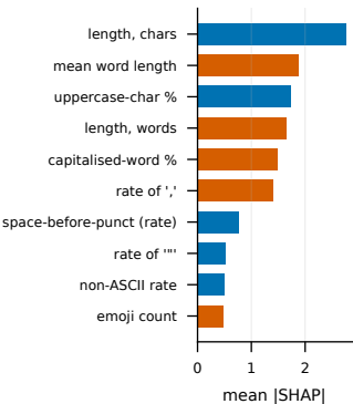
(a) DAIGT V2
