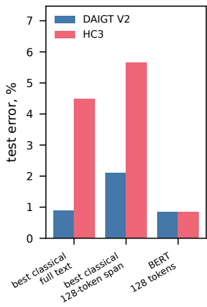
(d) Matched text budget
