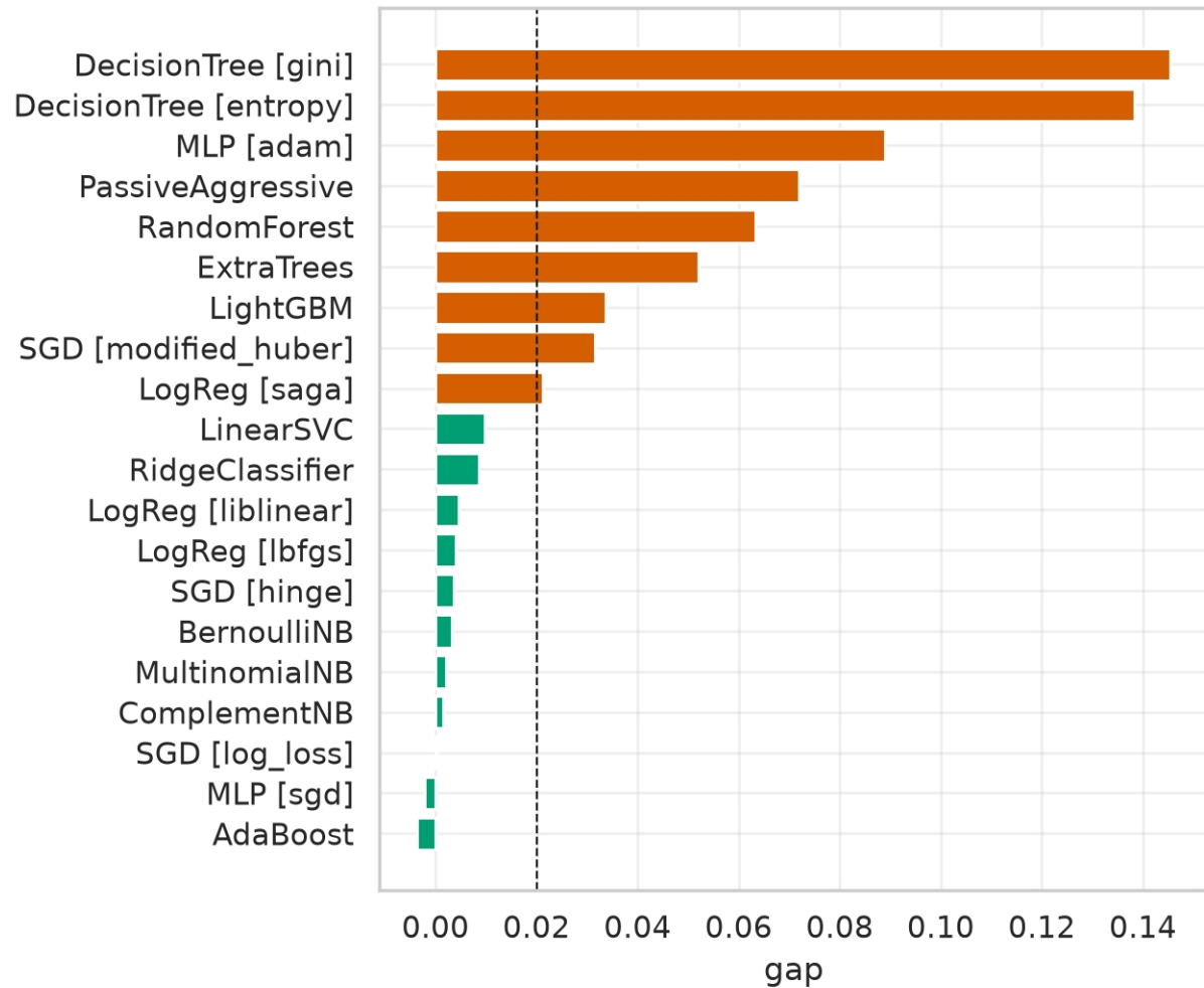
HC3: train F1 minus test F1
