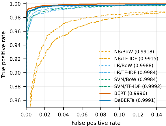
(a) DAIGT V2, detail
