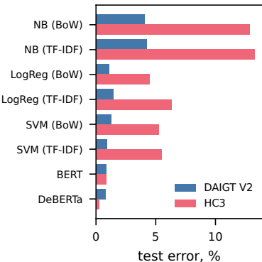
(d) Matched text budget
