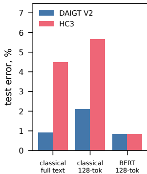
(d) Matched text budget
