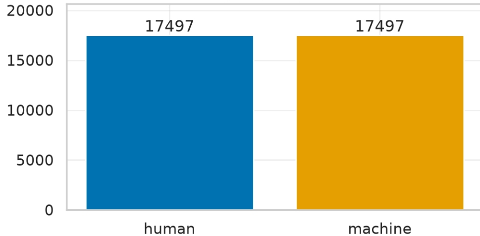
DAIGT V2
