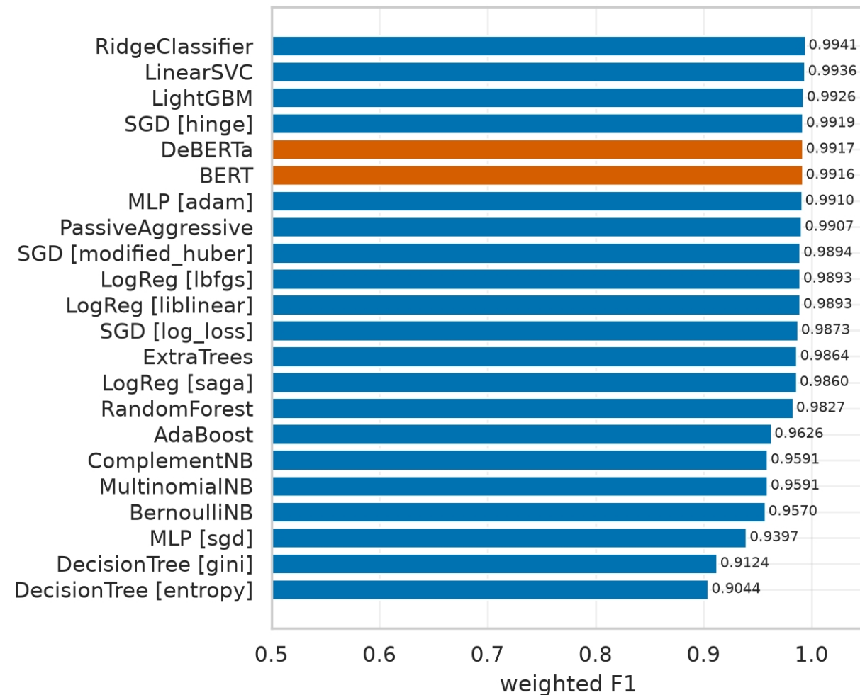
DAIGT V2
