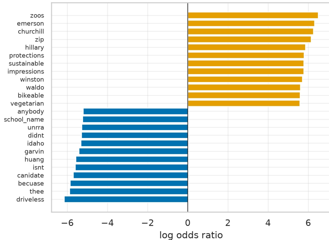
DAIGT V2
