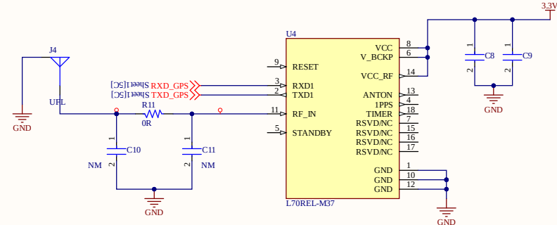
GPS
