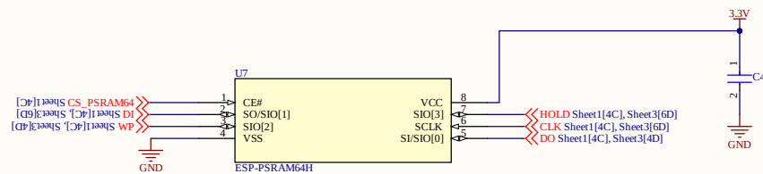
ESP32-S3 PSRAM64
