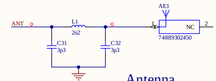
Antenna
