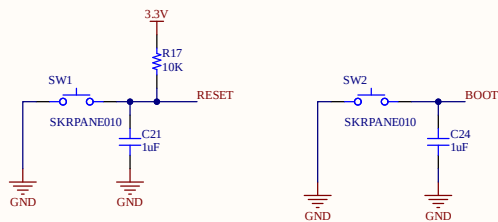
RESET
