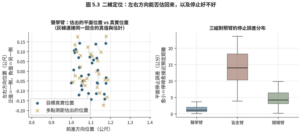
圖 5.3 二維定位：估出的平面位置與真實位置（左），三組對照臂的平面停止誤差（右）
