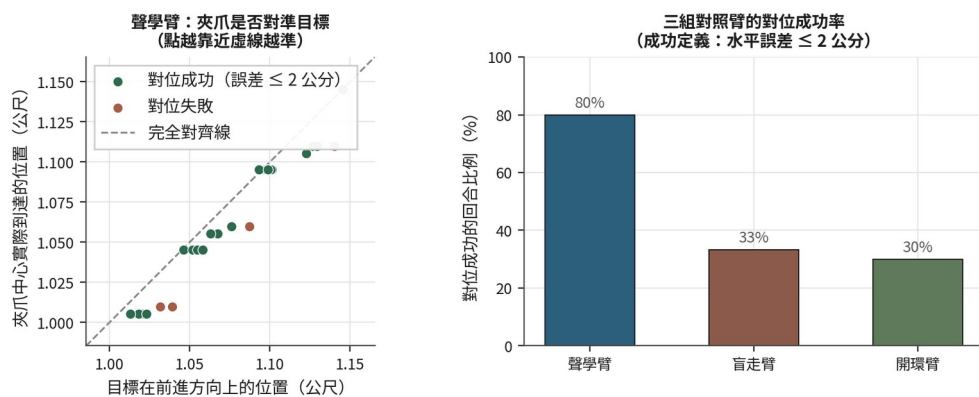
圖 5.2 夾取對位結果（走廊遠端修正後的正式複驗）
