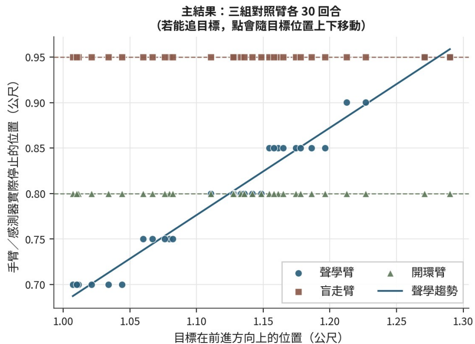
圖 5.1 閉環接近主結果：停止位置是否跟著目標走
