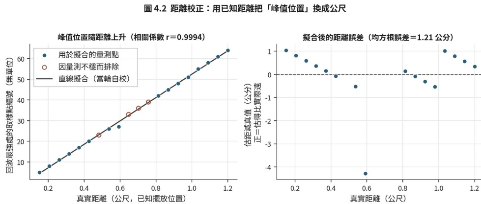
圖 4.2 距離校正：峰值位置對已知距離的直線擬合，以及估距誤差（公分）
