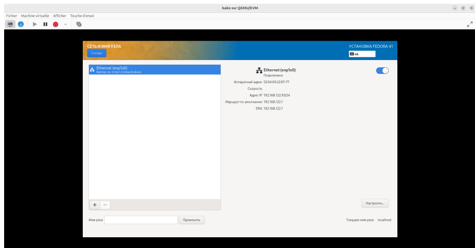
Figure 6: Настройка сети
