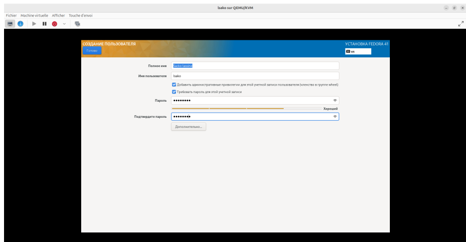
Figure 7: Создание пользователя
