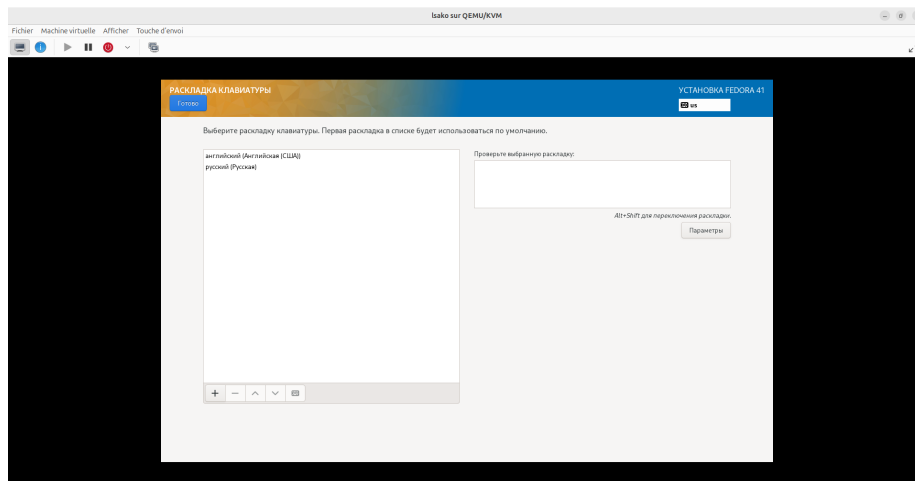
Figure 2: Раскладка клавиатуры
