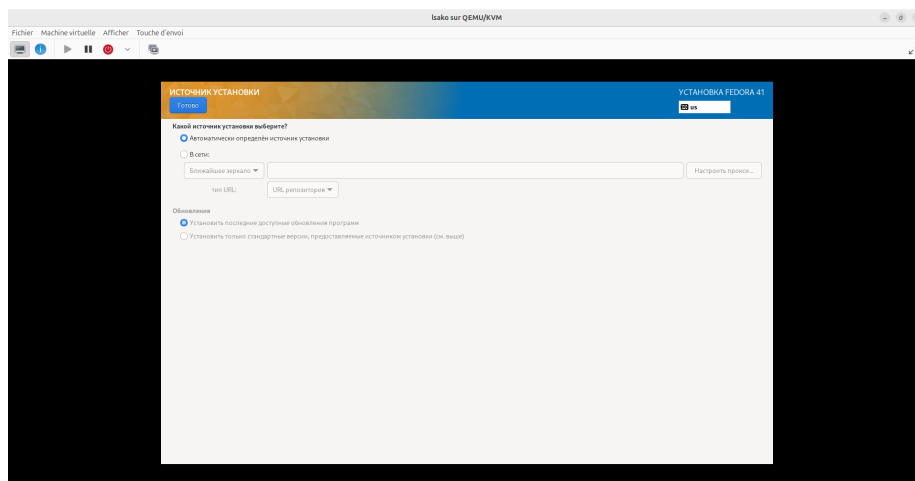
Figure 3: Источник установки
