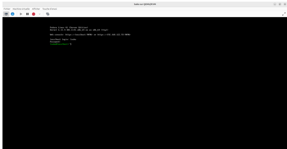
Figure 8: Экран входа
