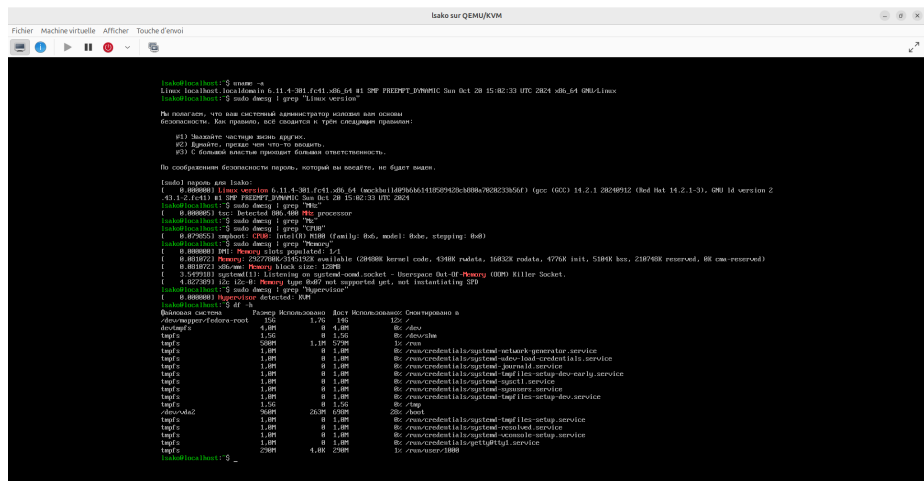
Figure 9: Терминал
