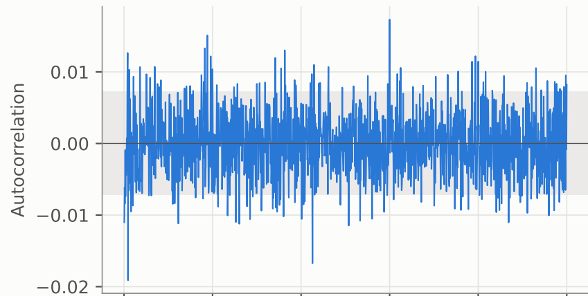
EUR/USD: absolute returns
