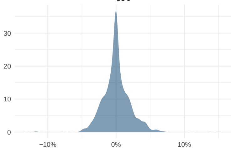
SPY
