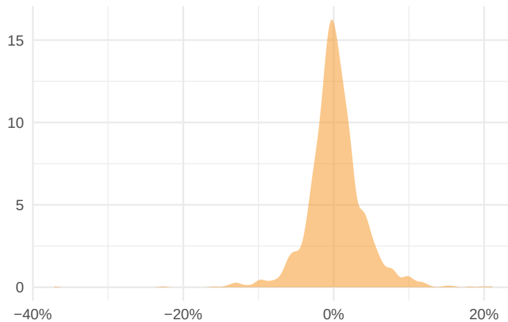
BTC
