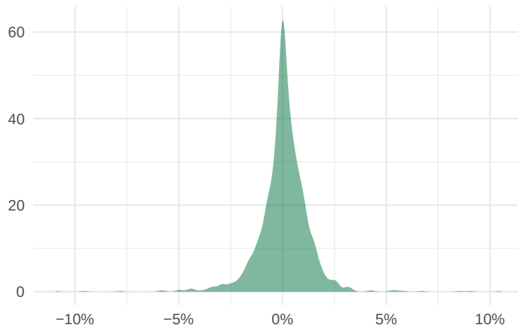
SPY
