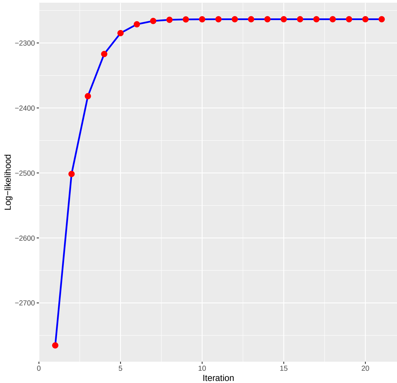
EM Convergence
