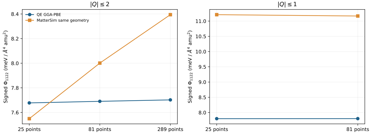
图 12: 固定宽窗（左）与中心窗（右）内，QE PBE 和同构型 MatterSim 的有符号四阶系数随位移采样步长变化。
