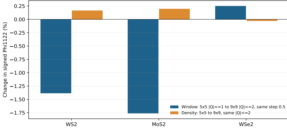
图 11: 将窗口变化与固定窗口下的采样密度变化分开展示。蓝色包含 |Q| \leq 1 \rightarrow 2 的窗口效应；橙色只改变 |Q| \leq 2 内的步长。
