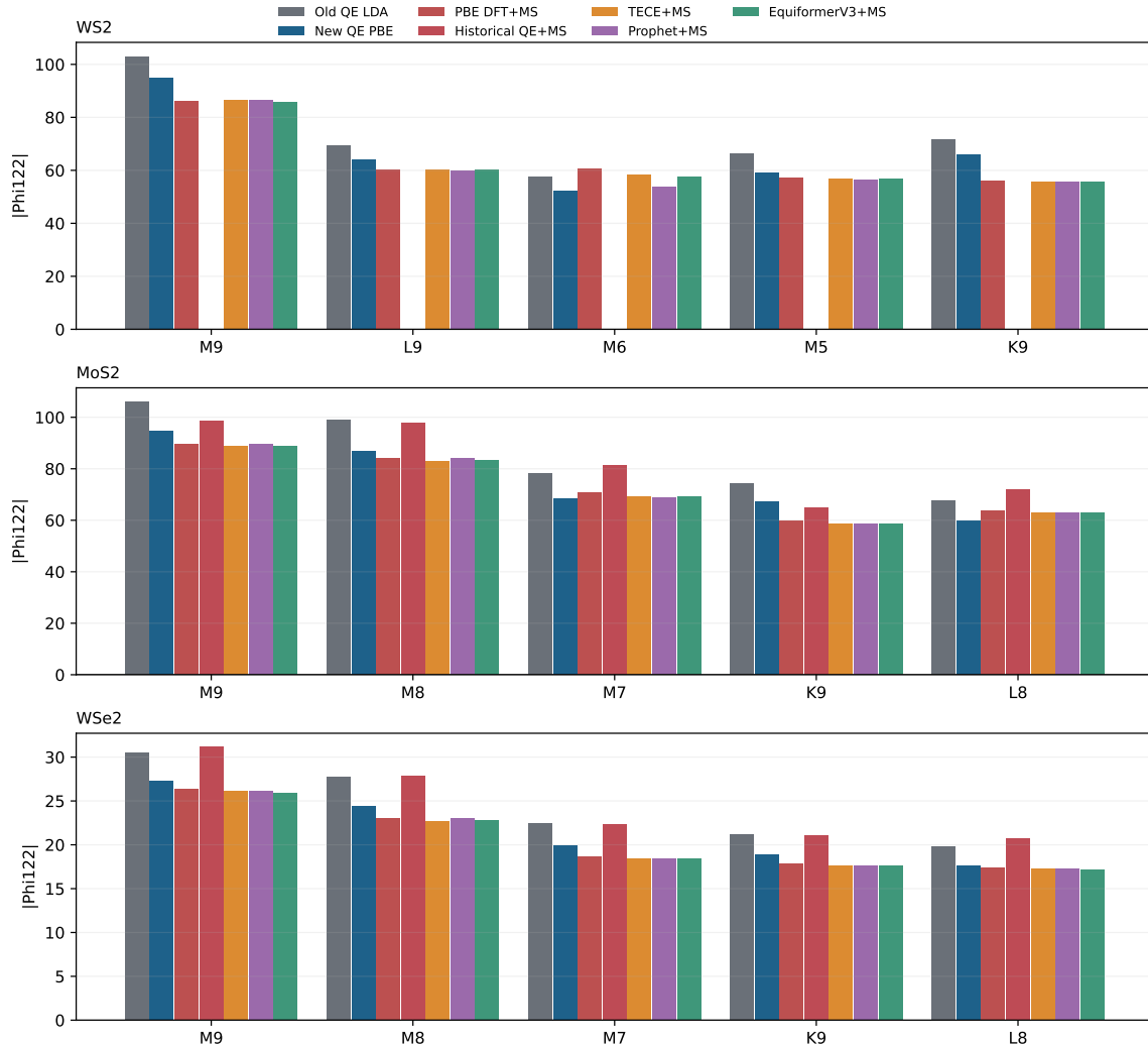
图 3: 十五个固定通道的三阶强度并列比较; 各材料五个通道分别排序展示。增加新 PBE DFT+MS 与旧 QE+MS 基线, 全部采用单位范数坐标; WS 2 历史基线缺失。参考由 LDA 转至 PBE 后, 首通道差距明显缩小。
