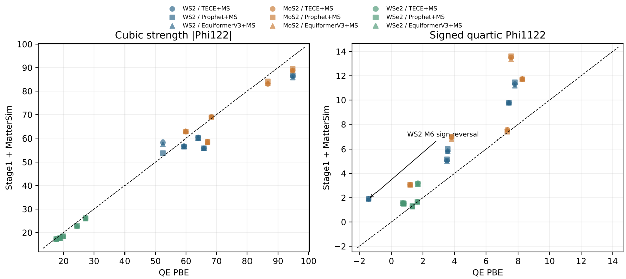
图 7: 三阶强度 (左) 与有符号四阶 (右) 相对 PBE 的散点。每种材料五对、每对三条 Stage1 路线; 虚线为完全一致。
