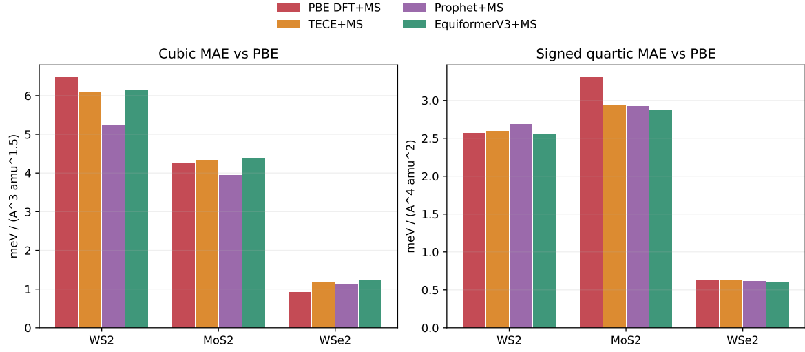
图 5: 在同一新 PBE 参考下比较新 DFT 模式基线与三条全 MLFF 路线; 全部比较最终物理通道的三阶强度和有序四阶。
