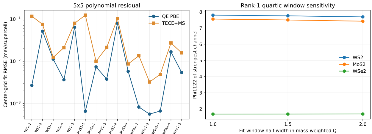
图 10: 左：每个通道中心拟合残差；右：每材料最强通道四阶值随窗口扩大而变化。低残差与低窗口敏感性是不同的检验。
