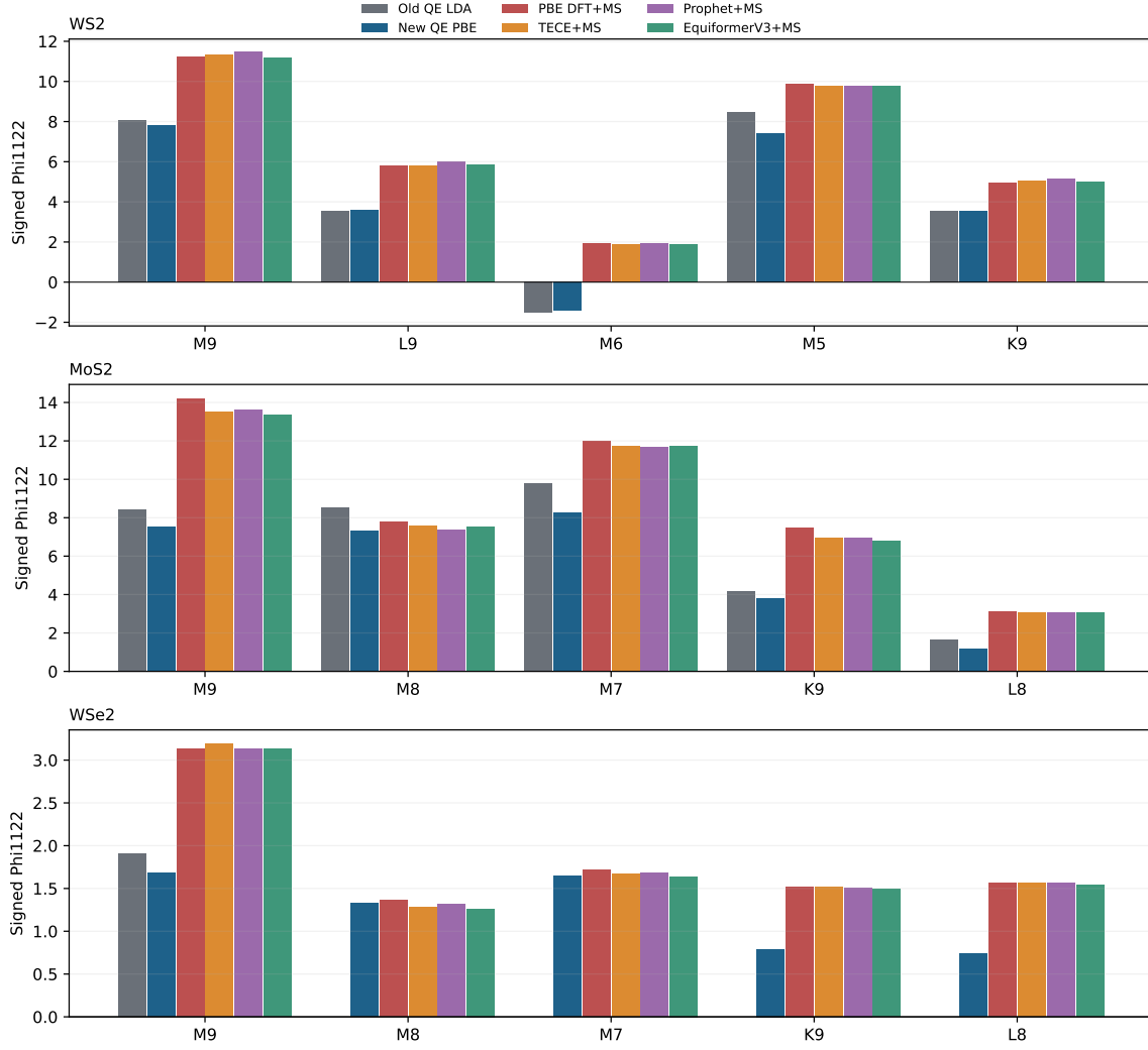
图 6: 有符号四阶导数对比; WS 2 的 M6 通道显示参考和 MLFF 势能面的实质性变号。
