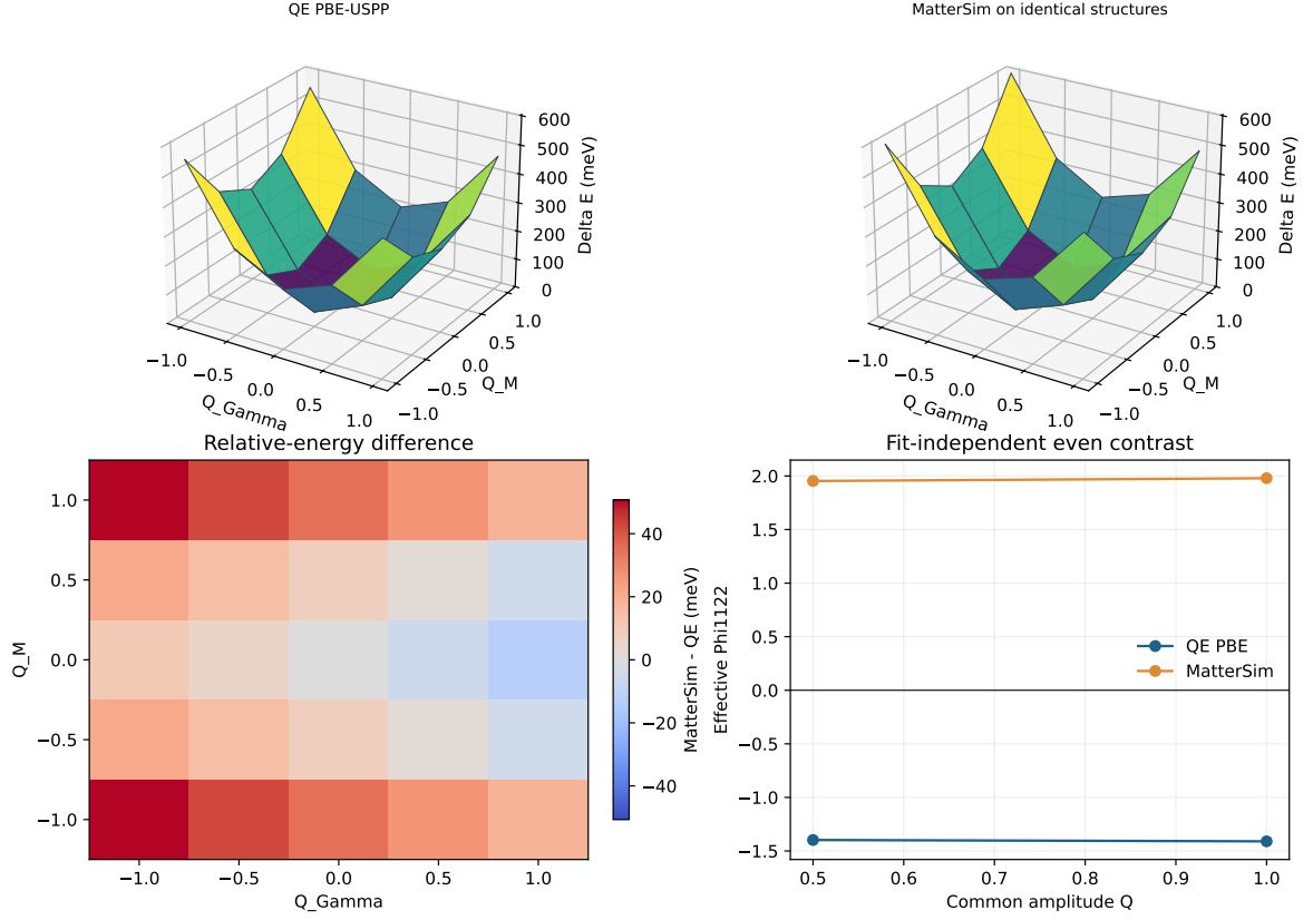
图 8: WS 2 M6 在相同 25 个构型上的 QE PBE 与 MatterSim 二维势能面、相对能差及拟合无关的偶混合对比。三维曲面的总体相似并不能保证微小四阶混合项同号。
