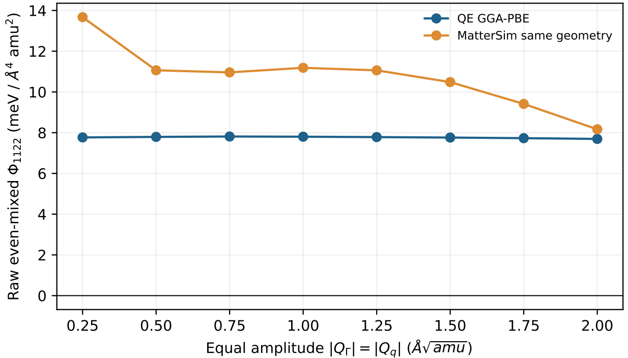
图 13: 不经过多项式拟合，由等幅四角点和坐标轴能量直接计算的有符号偶混合四阶估计。最小振幅的 MatterSim 值对浮点精度敏感。
