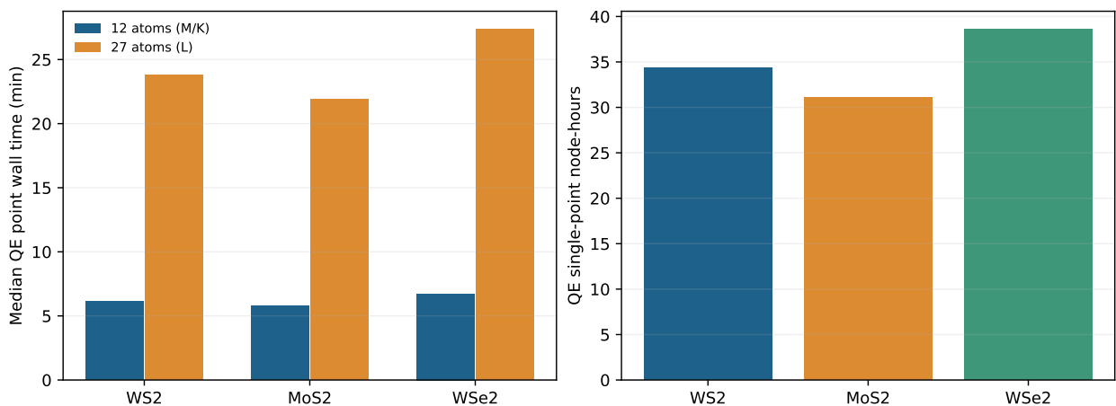
图 14: 左：12 与 27 原子超胞的 QE 单点中位墙钟；右：各材料 193 个单点的累计节点时。
