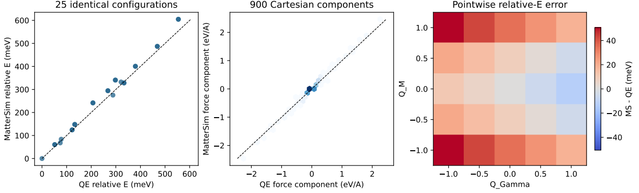
图 7: 同一 25 个 \text{WS}_2 PBE 构型的相对能量、900 个力分量及逐点相对能量差；仅此对照固定了所有原子坐标。
