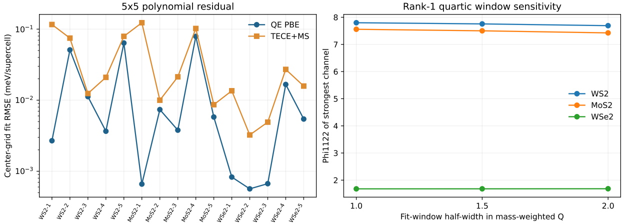
图 8: 左：每个通道中心拟合残差；右：每材料最强通道四阶值随窗口扩大而变化。低残差与低窗口敏感性是不同的检验。
