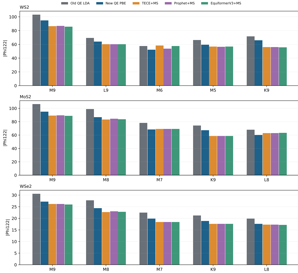
图 3: 十五个固定通道的三阶强度并列比较; 各材料五个通道分别排序展示。参考由 LDA 转至 PBE 后, 首通道差距明显缩小。
