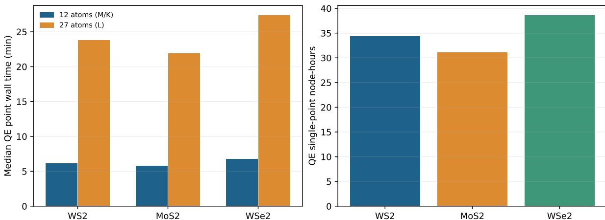
图 10: 左：12 与 27 原子超胞的 QE 单点中位墙钟；右：各材料 193 个单点的累计节点时。
