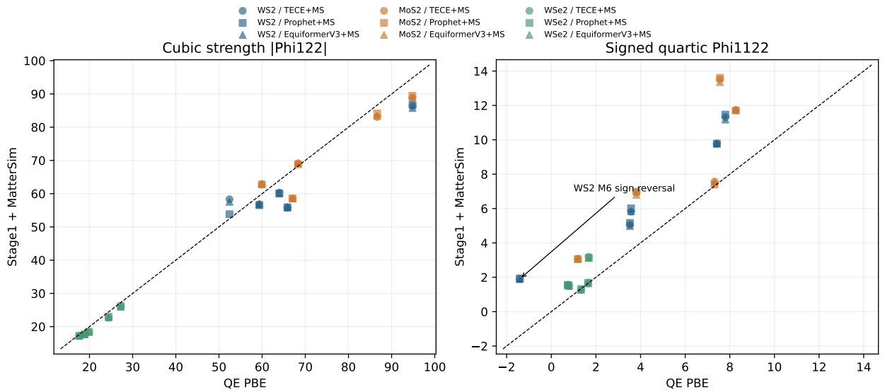
图 5: 三阶强度 (左) 与有符号四阶 (右) 相对 PBE 的散点。每种材料五对、每对三条 Stage1 路线; 虚线为完全一致。
