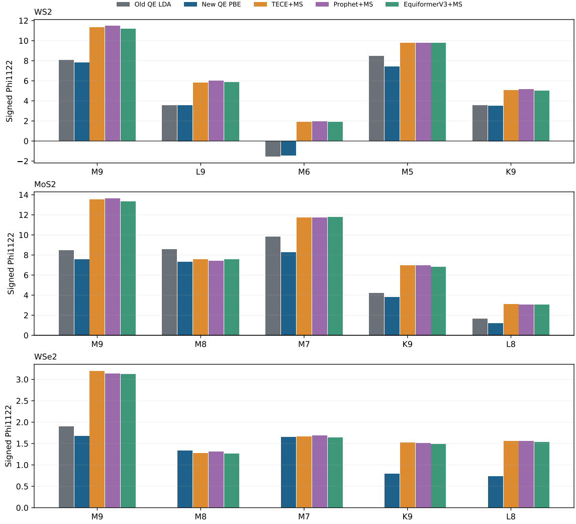
图 4: 有符号四阶导数对比; WS 2 的 M6 通道显示参考和 MLFF 势能面的实质性变号。
