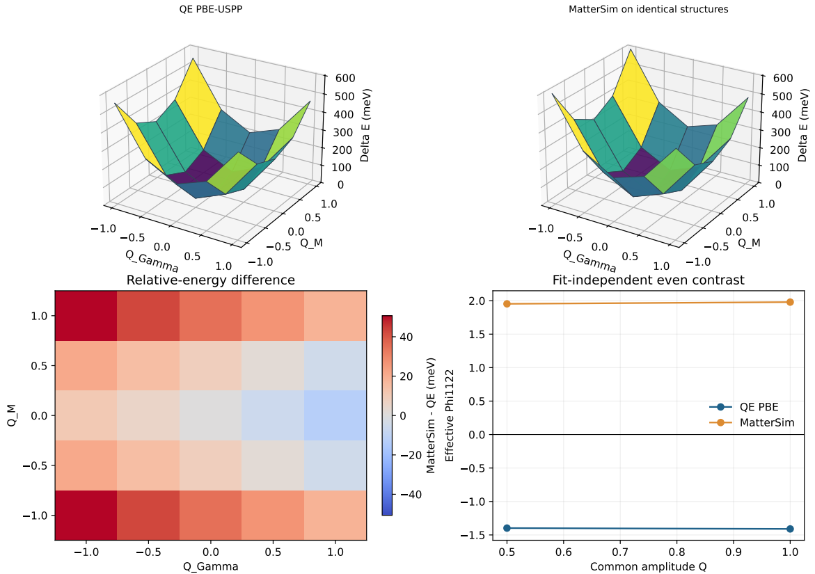
图 6: WS 2 M6 在相同 25 个构型上的 QE PBE 与 MatterSim 二维势能面、相对能差及拟合无关的偶混合对比。三维曲面的总体相似并不能保证微小四阶混合项同号。
