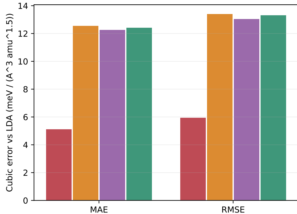
MoS2
