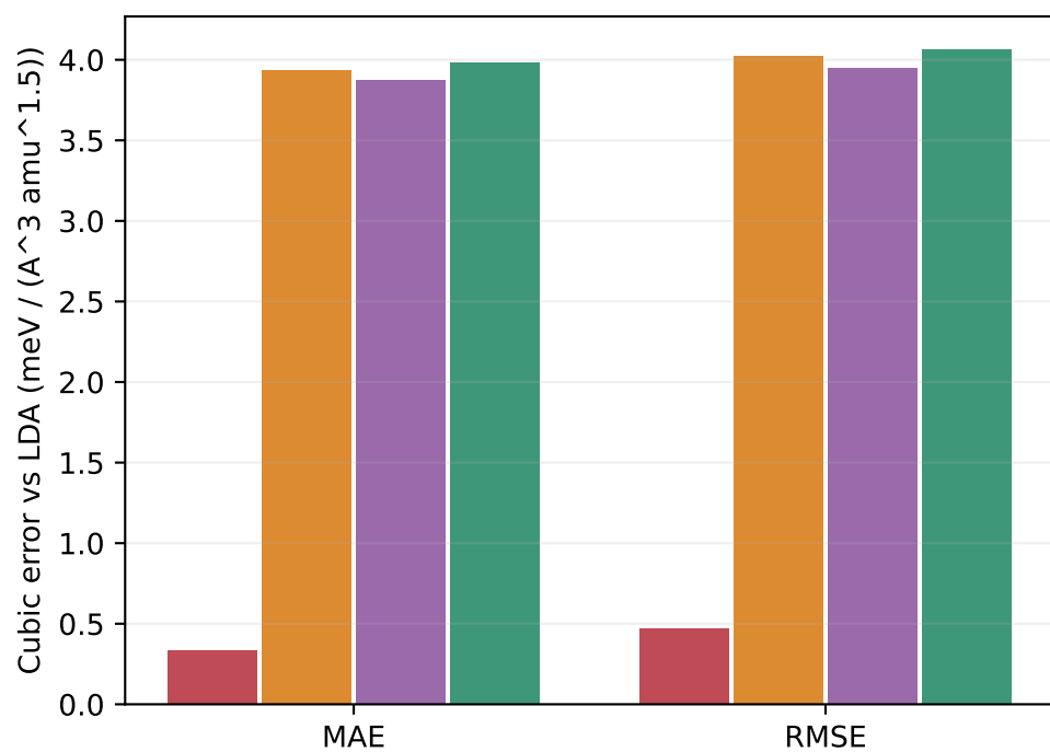
WSe2
