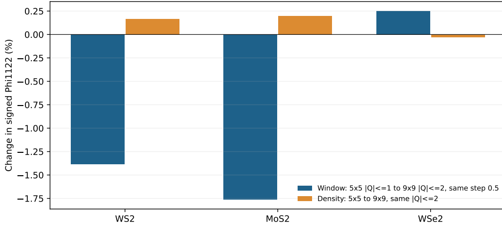
图 16: 将窗口变化与固定窗口下的采样密度变化分开展示。蓝色包含 |Q| \leq 1 \rightarrow 2 的窗口效应；橙色只改变 |Q| \leq 2 内的步长。
