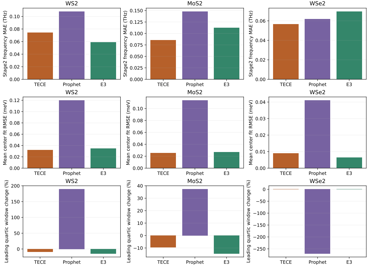
图 7: 全流程 Stage2 曲率频率误差、中心拟合残差及首通道四阶窗口变化。对应 Stage1 频率已由此前完整 6×6 比较给出。
