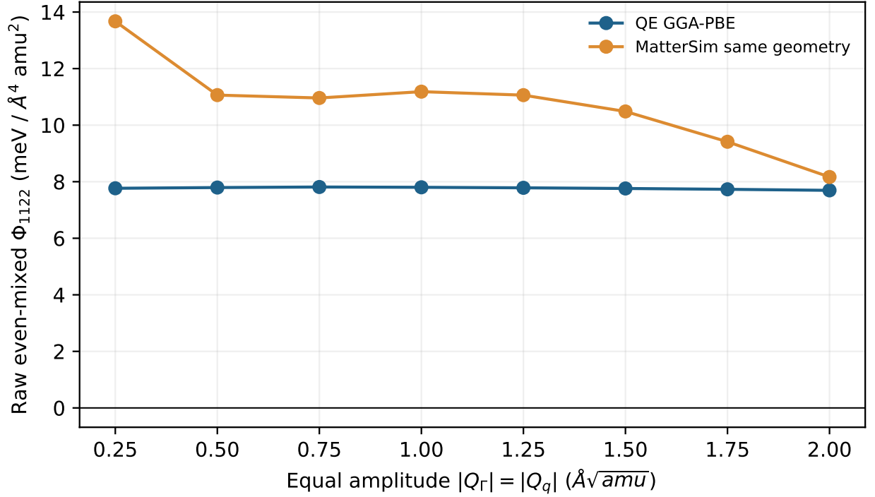
图 18: 不经过多项式拟合，由等幅四角点和坐标轴能量直接计算的有符号偶混合四阶估计。最小振幅的 MatterSim 值对浮点精度敏感。
