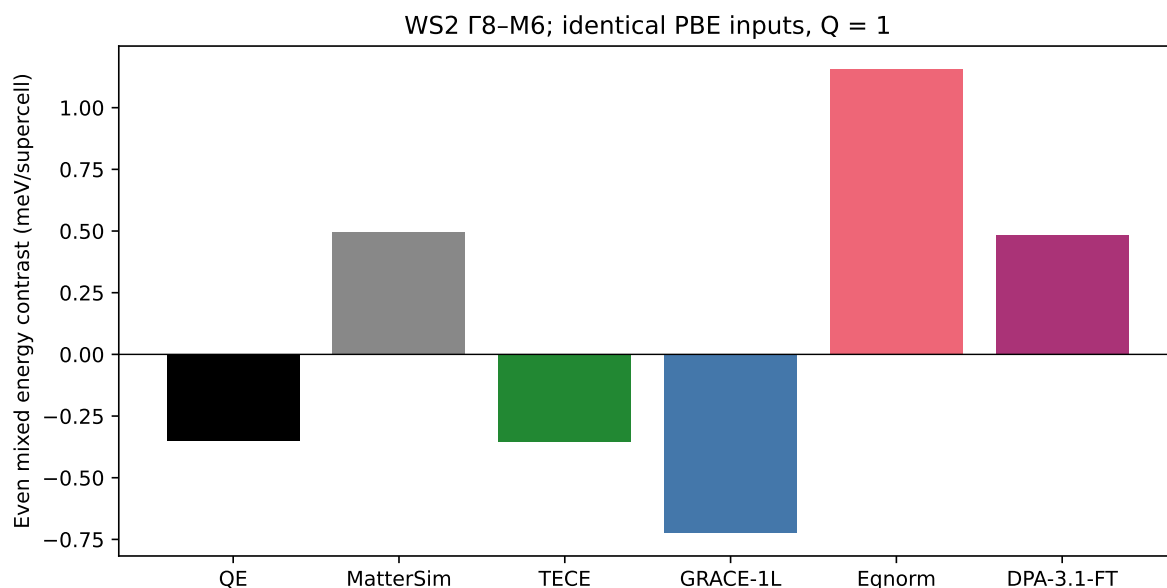
图 10: WS 2 \Gamma 8-M6 在 |Q_1| = |Q_2| = 1 的偶混合原始能量差。无需多项式拟合就能看到 MatterSim、Eqnorm、DPA 给出的相互作用方向与 QE 相反；TECE 接近 QE，GRACE 方向正确但幅度偏大。该量包含更高偶阶项，不等于单独的四阶 Taylor 系数。
