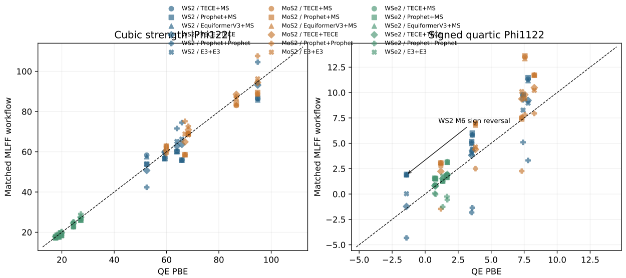
图 12: 三阶强度 (左) 与有符号四阶 (右), 包含 MatterSim 混合路线和三条同模型全流程相对 PBE 的散点。每种材料五对、每对三条 Stage1 路线; 虚线为完全一致。
