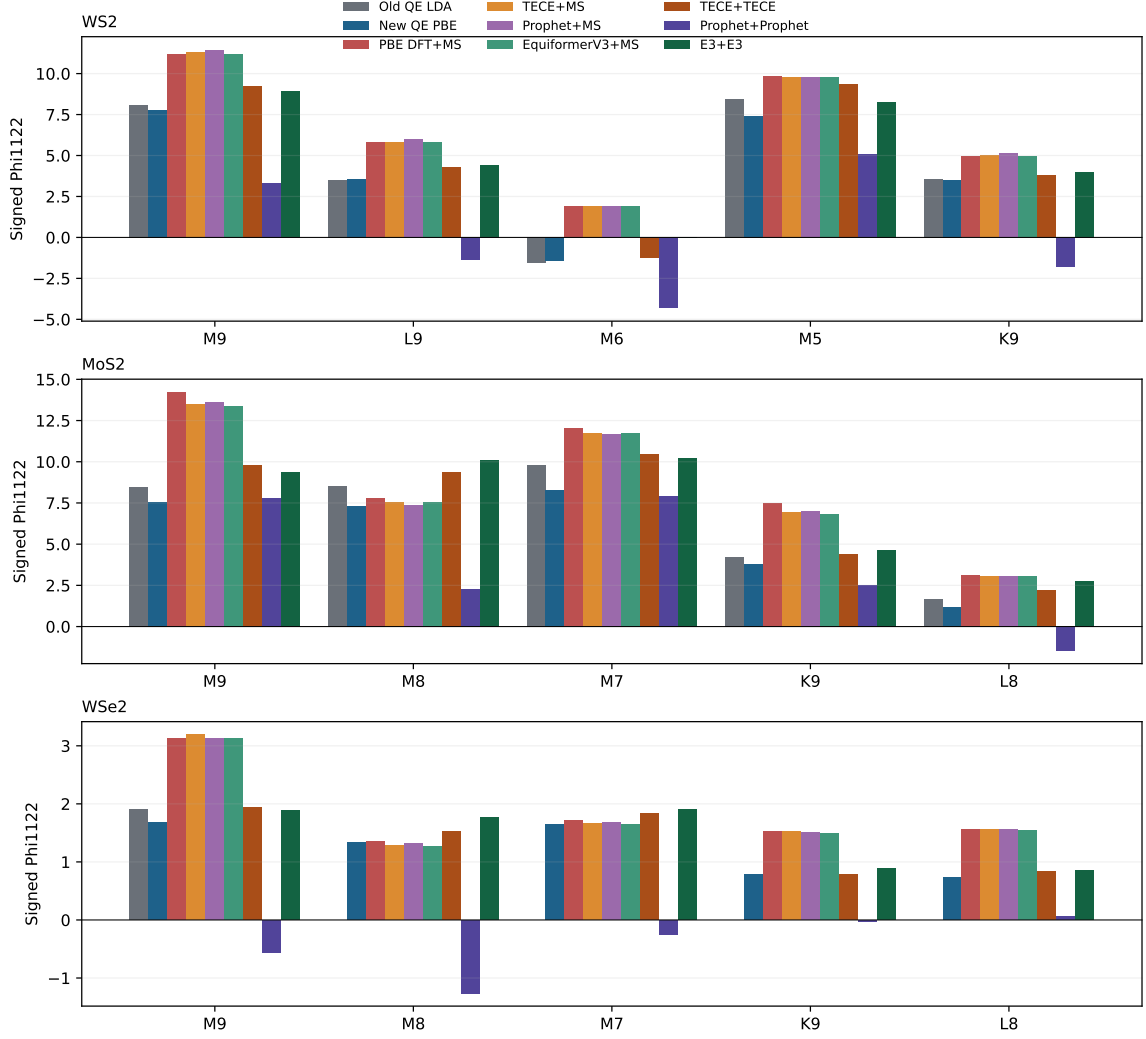
图 11: 有符号四阶导数对比; \text{WS}_2 的 M6 通道显示参考和 MLFF 势能面的实质性变号。
