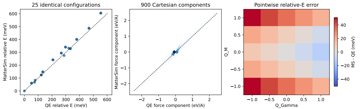
图 14: 同一 25 个 WS 2 PBE 构型的相对能量、900 个力分量及逐点相对能量差；仅此对照固定了所有原子坐标。
