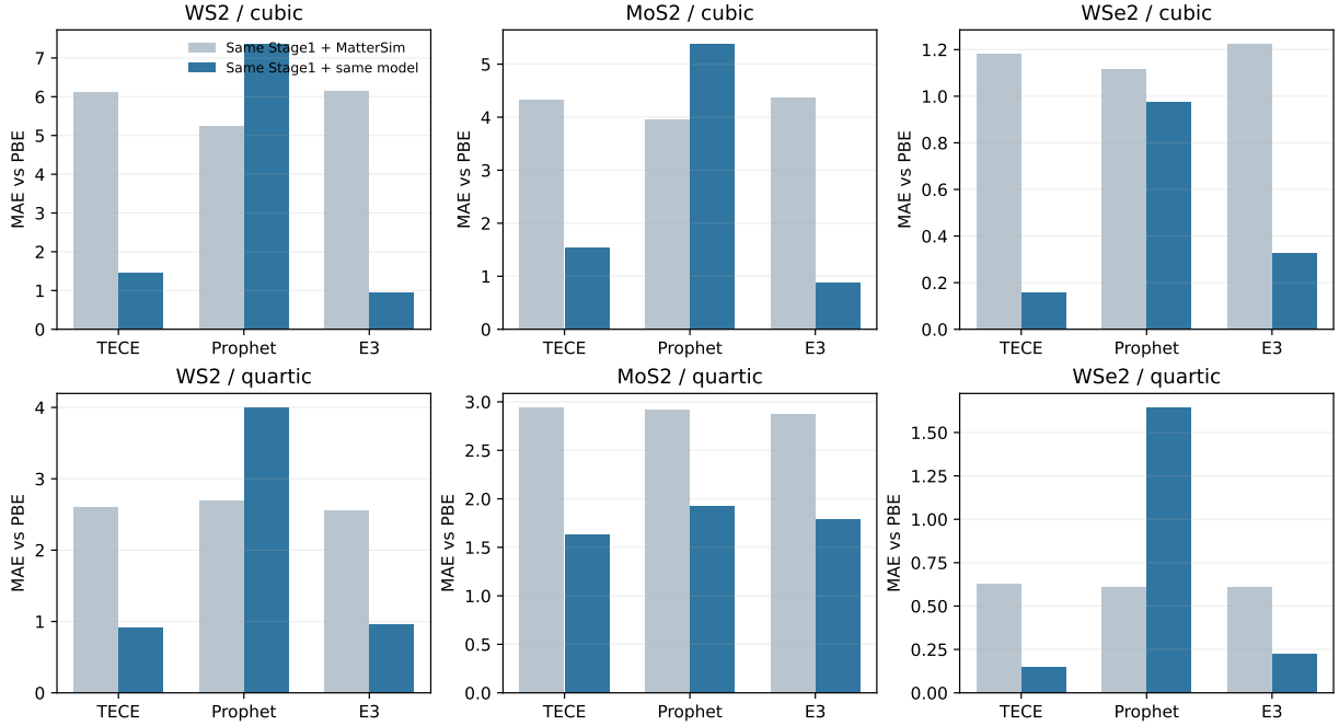
图 6: 复用完全相同的 Stage1 结构和模式后, 更换 Stage2 对三四阶 MAE 的影响。每材料仅五个既定强通道, 不能推广为未筛选的全部材料误差。
