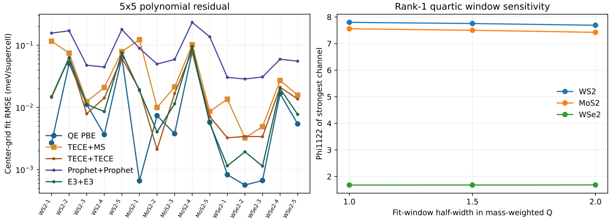
图 15: 左：每个通道中心拟合残差；右：每材料最强通道四阶值随窗口扩大而变化。低残差与低窗口敏感性是不同的检验。
