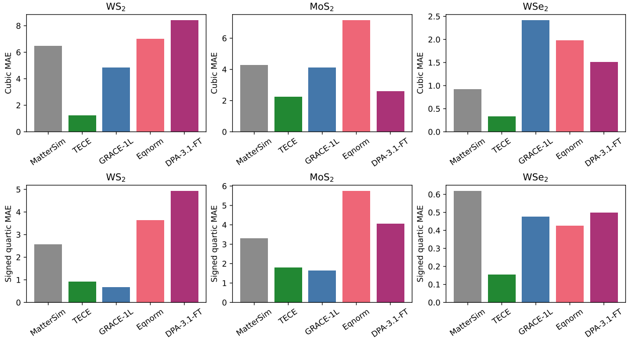
图 9: 固定同一 PBE DFT 结构和模态时, MatterSim、TECE 与三个小模型的三阶强度和有符号四阶 MAE。各材料五个通道, 排除了 Stage1 结构与模式的变化。
