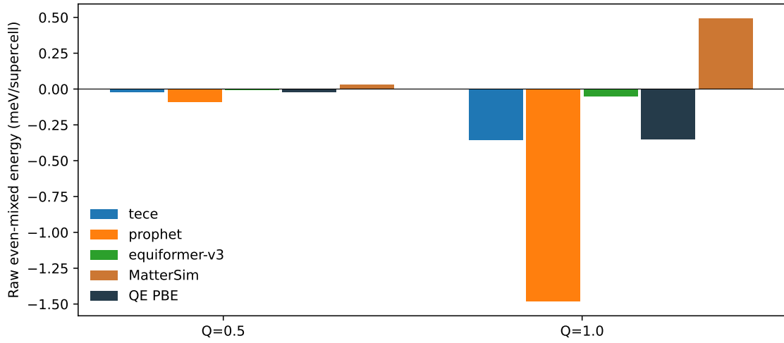
图 8: WS 2 \Gamma_8 -M6 固定 PBE 构型的偶混合能量差。直接由原始能量消去轴向项及奇次项，不经多项式拟合。
