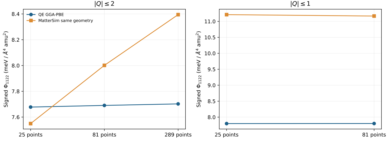
图 17: 固定宽窗（左）与中心窗（右）内，QE PBE 和同构型 MatterSim 的有符号四阶系数随位移采样步长变化。
