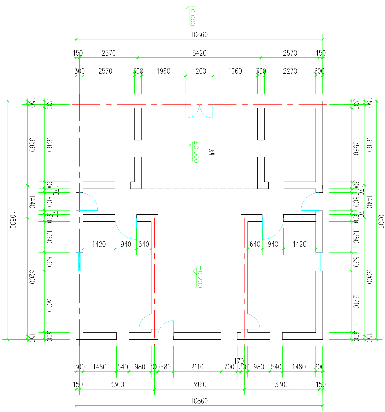
一层平面
