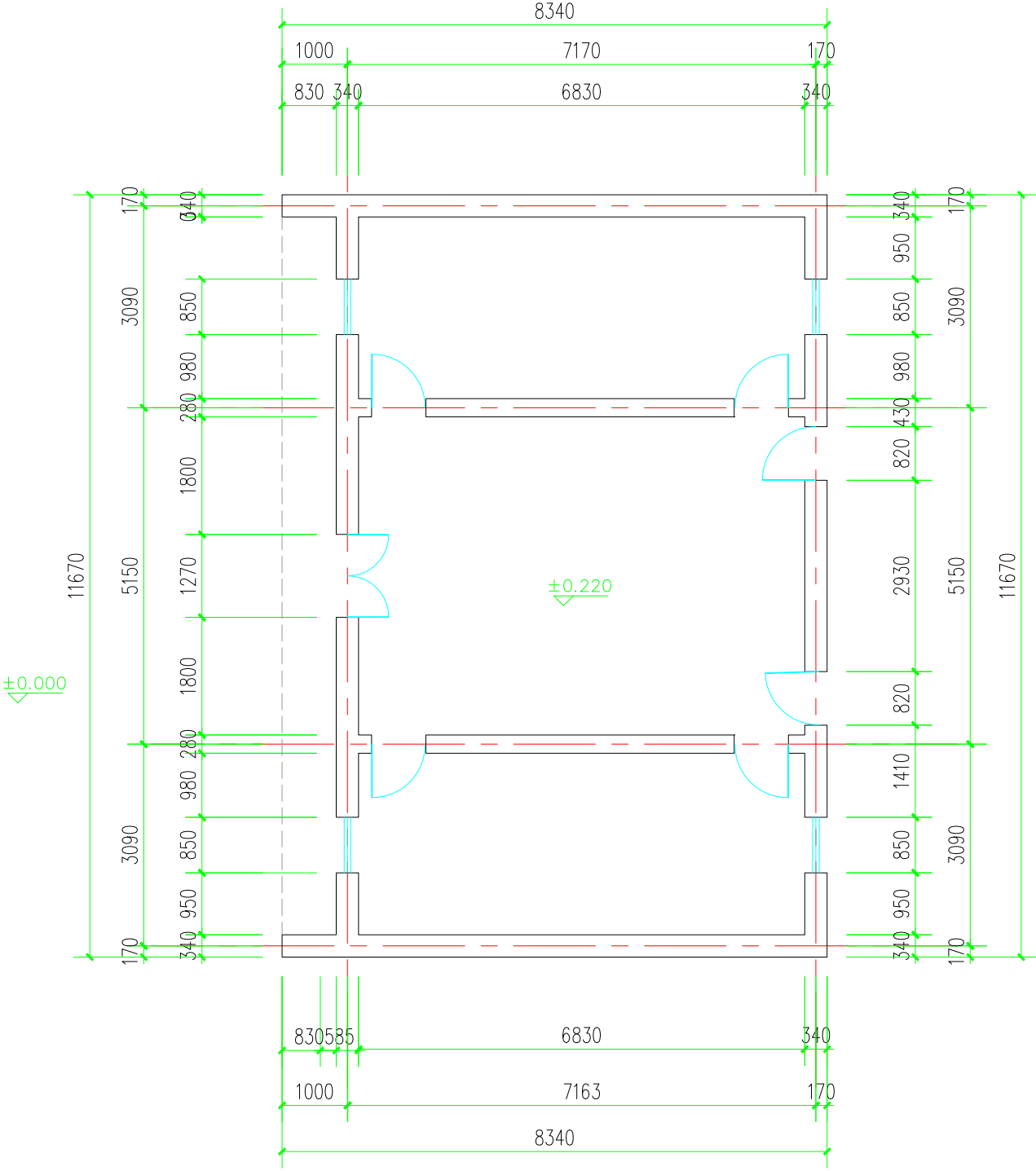
一层平面
