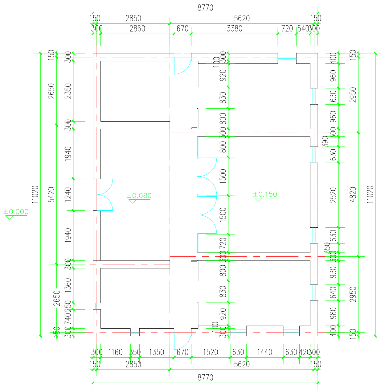
一层平面
