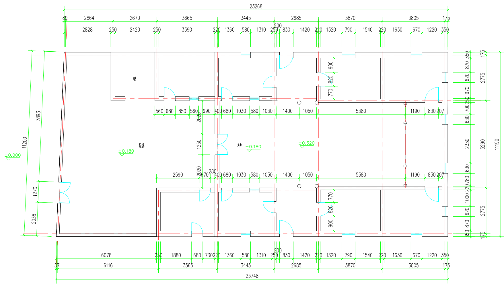
一层平面
